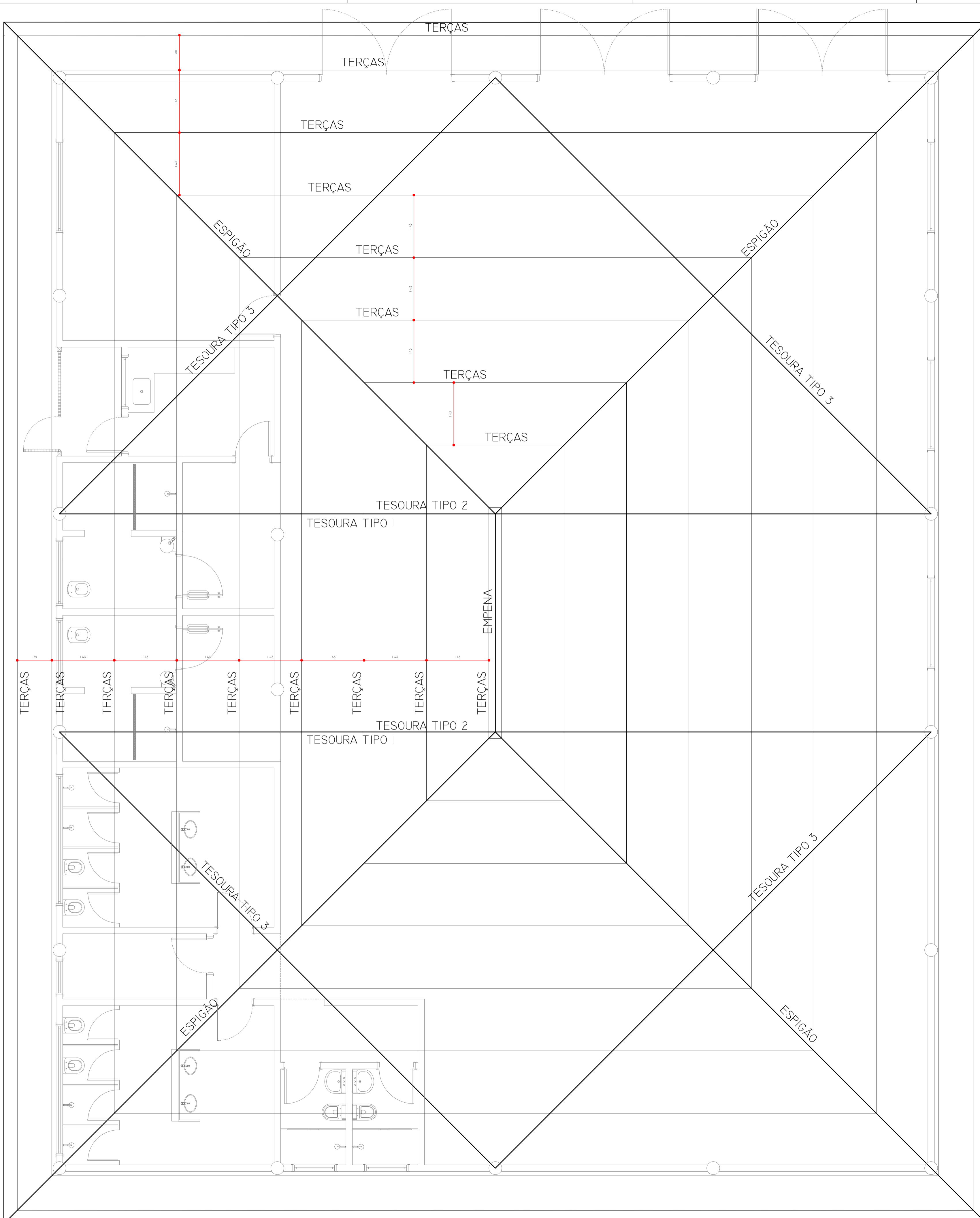
PLANTA DE COBERTURA ESC.: 1:50
