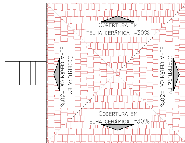
PLANTA DE COBERTURA ESC: 1/100
