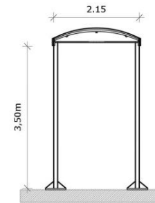
CORTE: Toldo A
