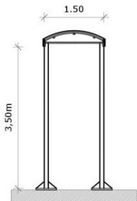
CORTE: Toldo B
