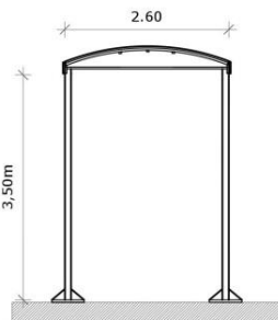
CORTE: Toldo B
