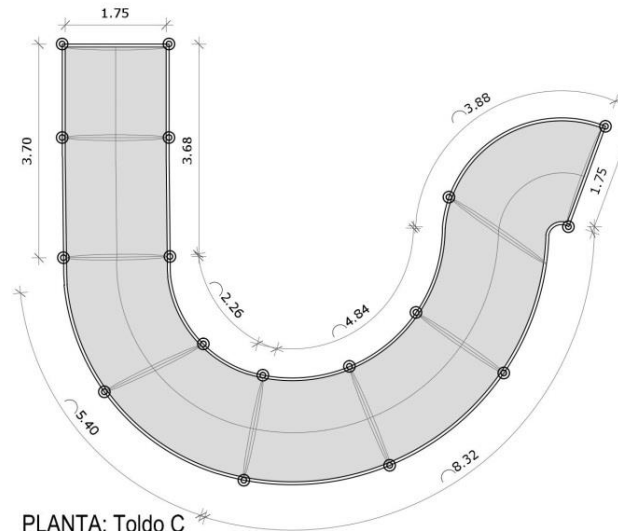
PLANTA: Toldo C
