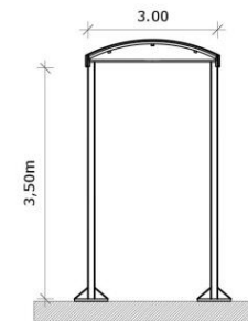
CORTE: Toldo A
