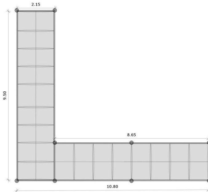
PLANTA:Toldo A
