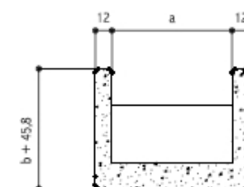
CORTE AA'
