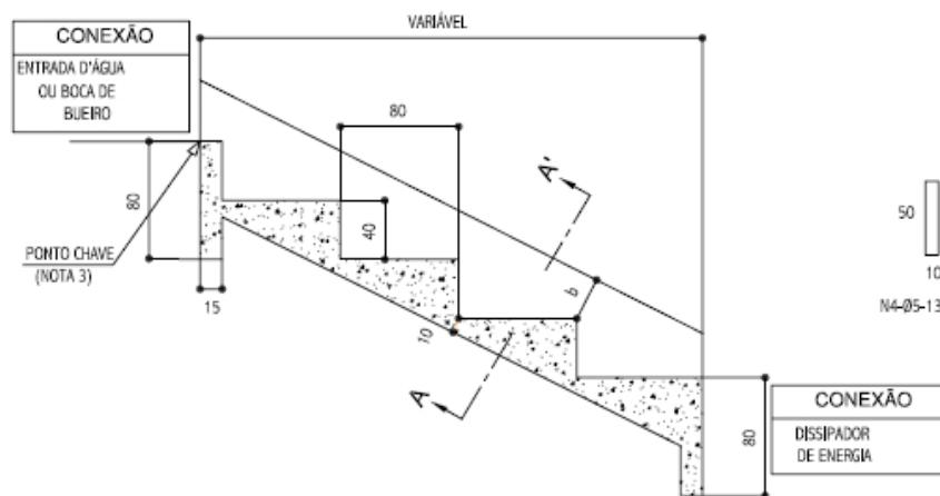
CORTE LONGITUDINAL
