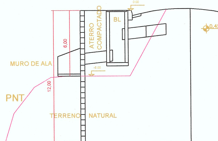
CORTE BB SEM ESC.
