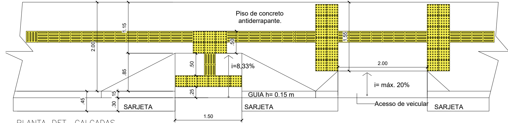
PLANTA DET. CALÇADAS Esc.: 1/50
