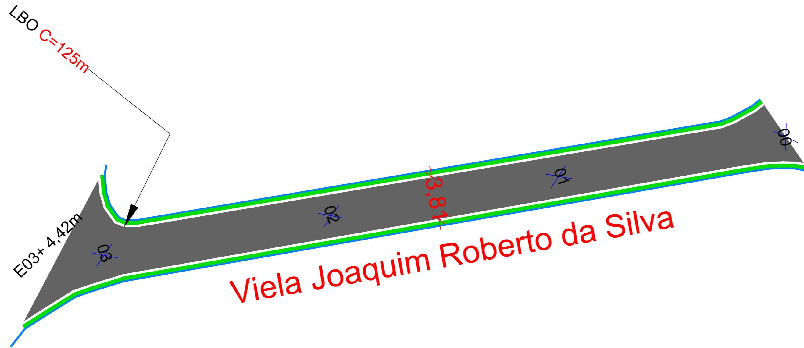
DETALHE 1 – GUIAS E SARJETAS / RECAPEAMENTO SEM ESCALA
