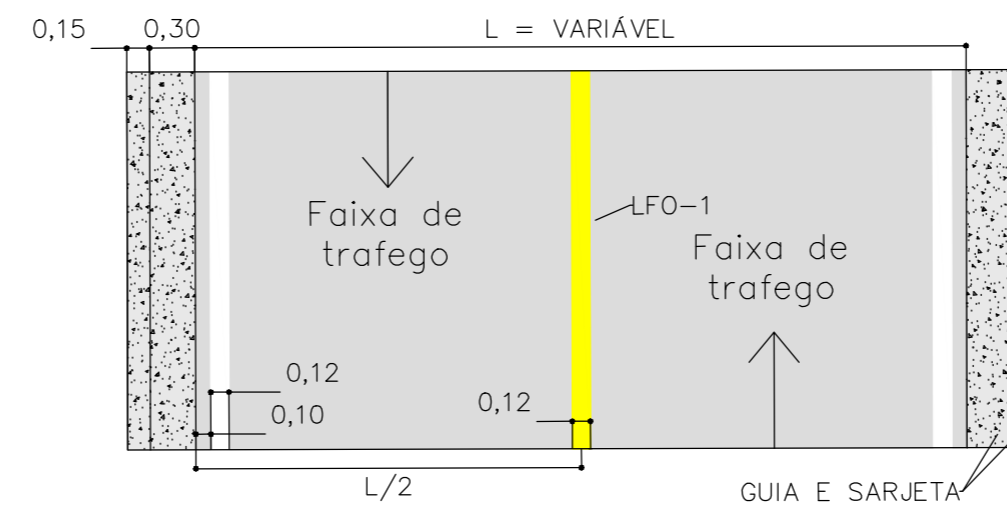
DETALHE 2 – SINALIZAÇÃO HORIZONTAL SEM ESCALA
