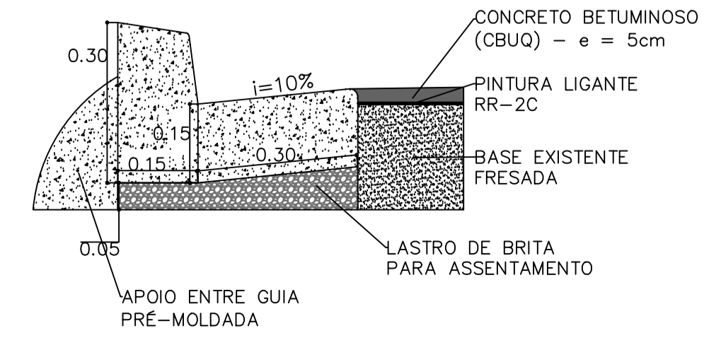
DETALHE 2 – GUIAS E SARJETAS / RECAPEAMENTO SEM ESCALA
