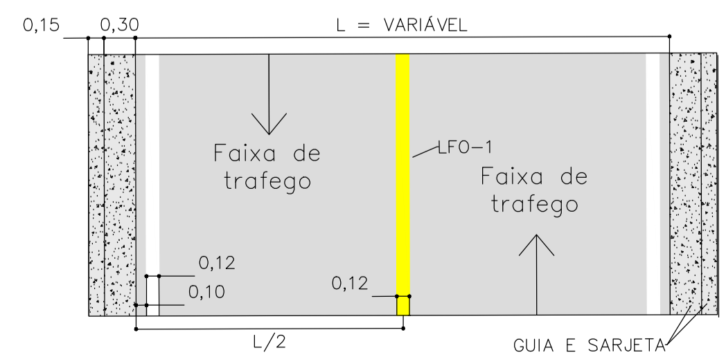
DETALHE 1 – SINALIZAÇÃO HORIZONTAL SEM ESCALA
