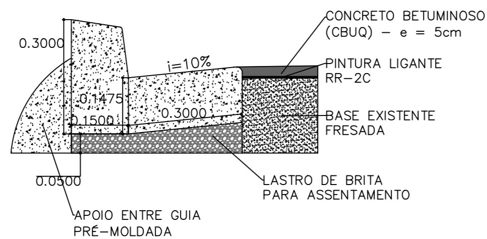
DETALHE 1 – GUIAS E SARJETAS / RECAPEAMENTO SEM ESCALA
