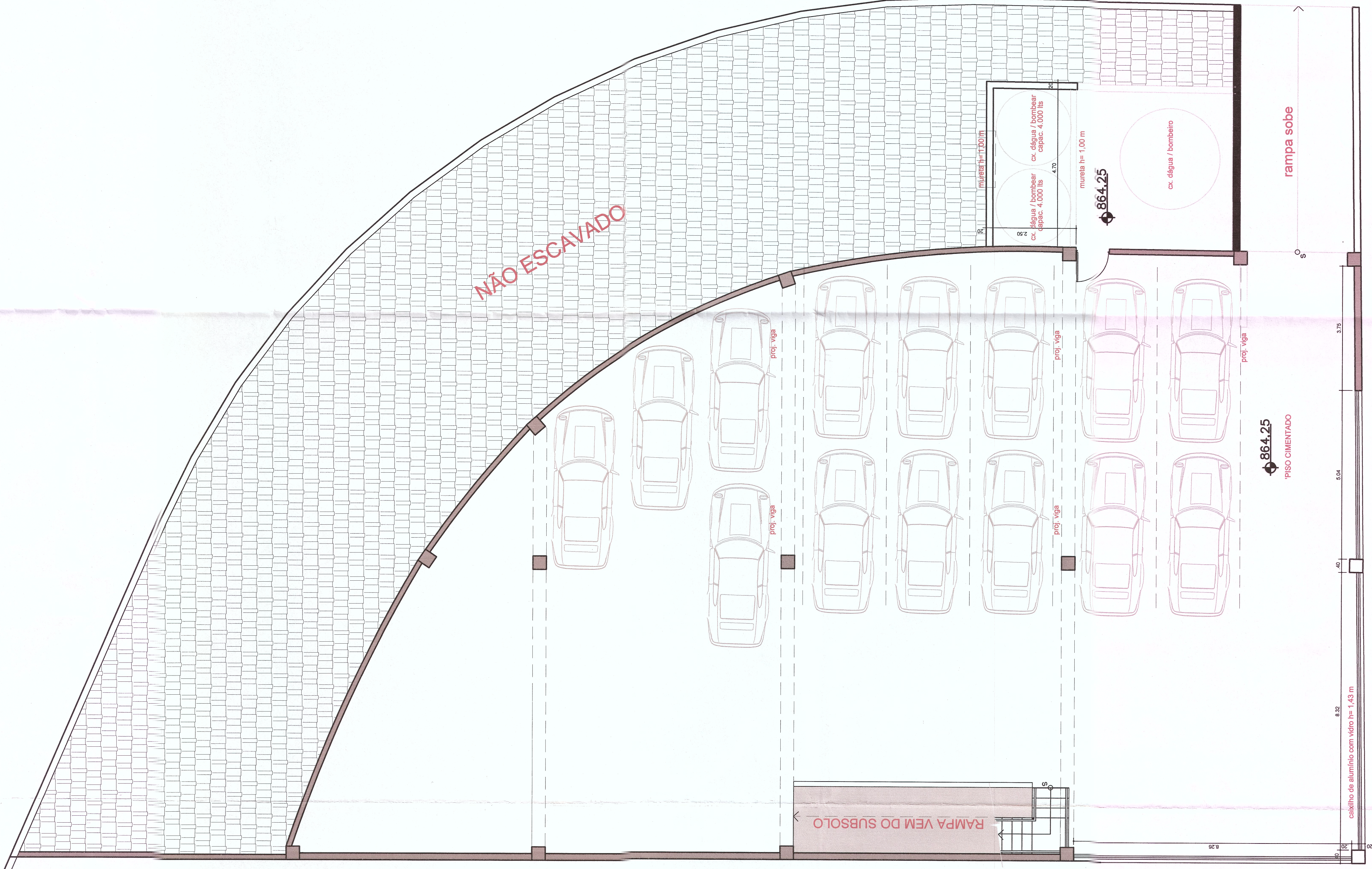
PLANTA SUBSOLO-ESTACIONAMENTO - NÍVEL +864.25 ESC. 1:75
