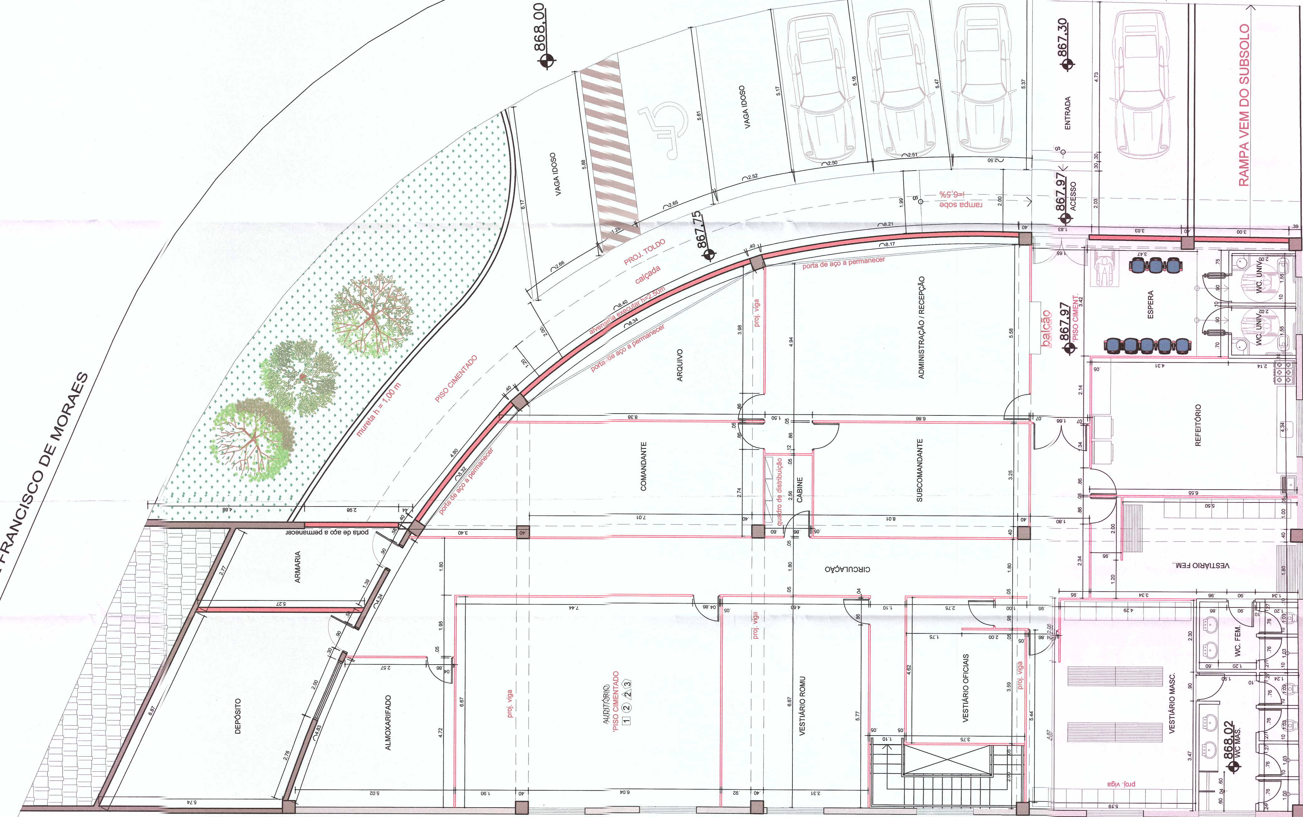
PLANTA LAY OUT - DIVISÓRIAS E MOBILIÁRIO- NÍVEL +867.97 ESC. 1:75
