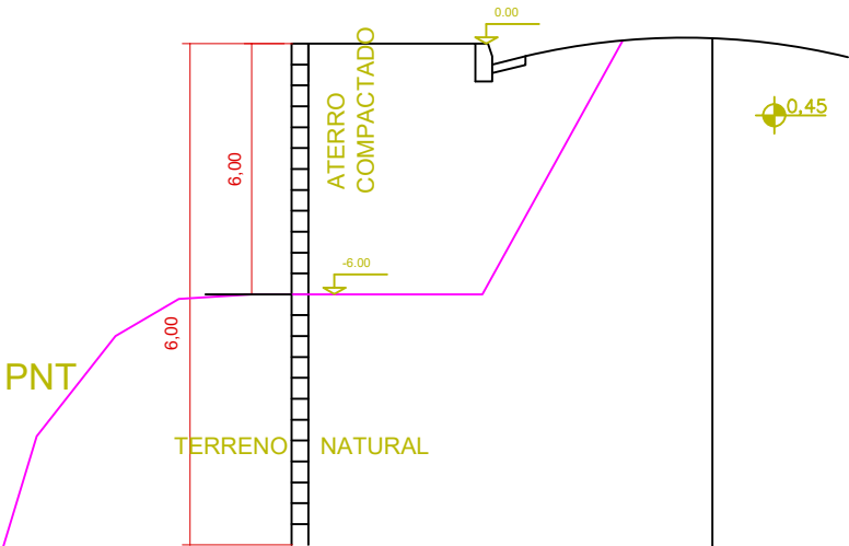
CORTE BB SEM ESC.
