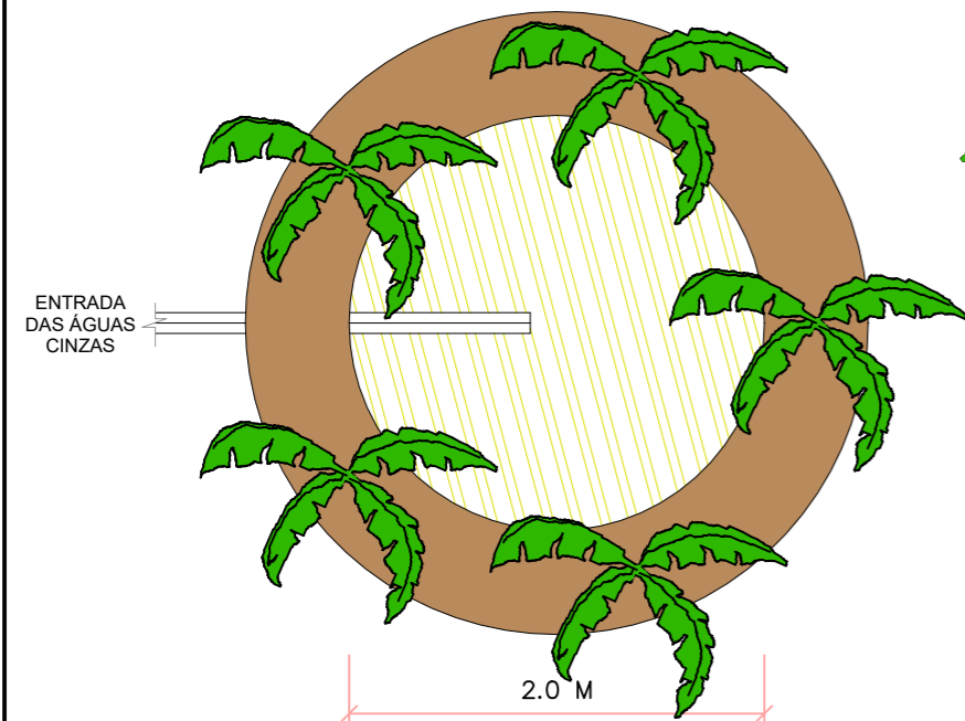
CÍRCULO DE BANANEIRAS - 5 PESSOAS SEM ESCALA
