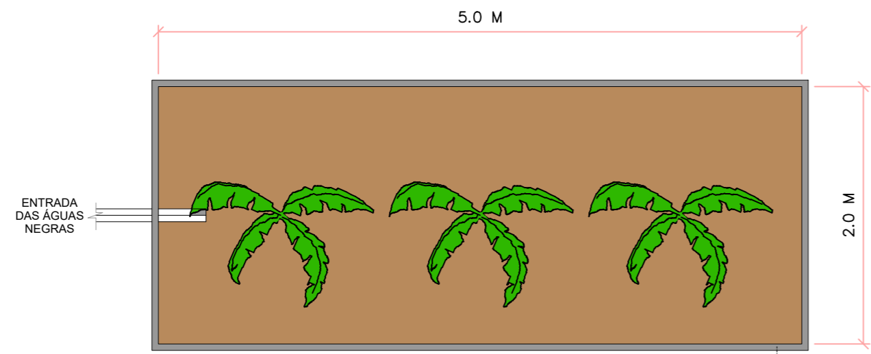
TANQUE DE EVAPOTRANSPIRAÇÃO (TEVAP) - 5 PESSOAS SEM ESCALA
