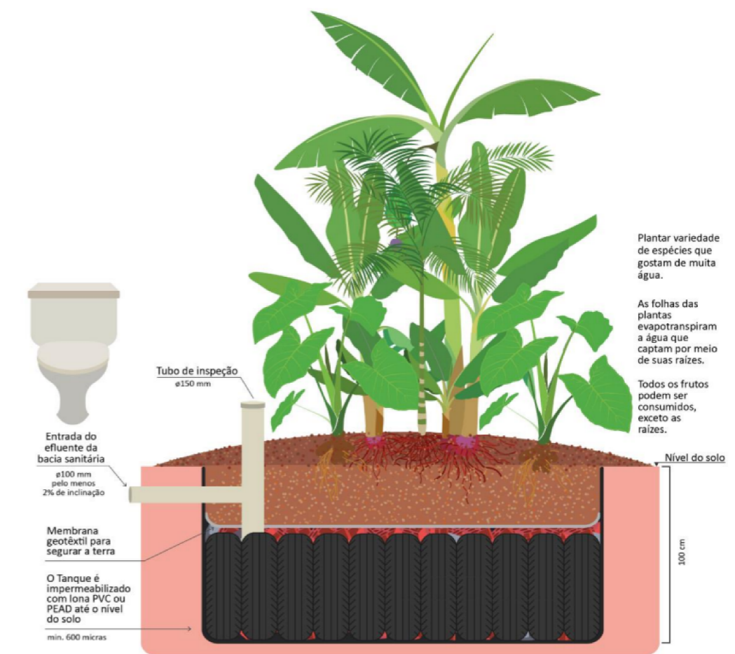
DETALHE LONGITUDINAL - TANQUE DE EVAPOTRANSPIRAÇÃO SEM ESCALA
