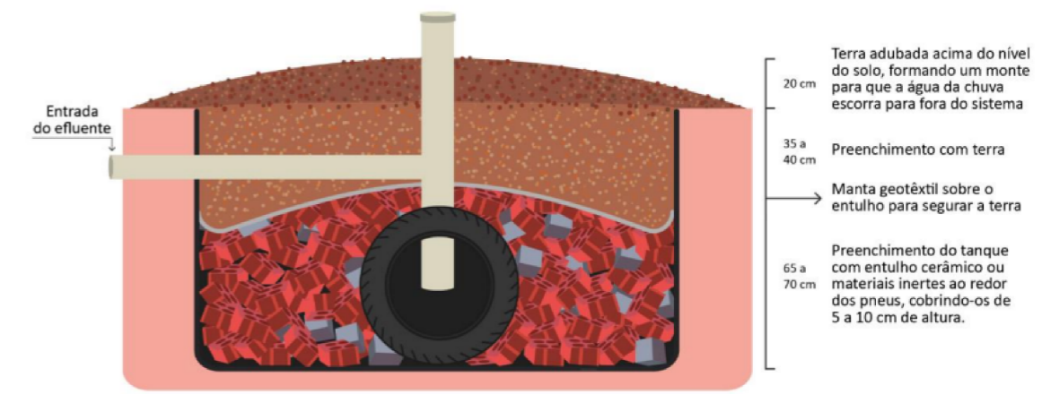
DETALHE TRANSVERSAL - TANQUE DE EVAPOTRANSPIRAÇÃO SEM ESCALA
