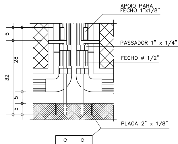
DETALHE 3 - FECHO INFERIOR SEM ESCALA
