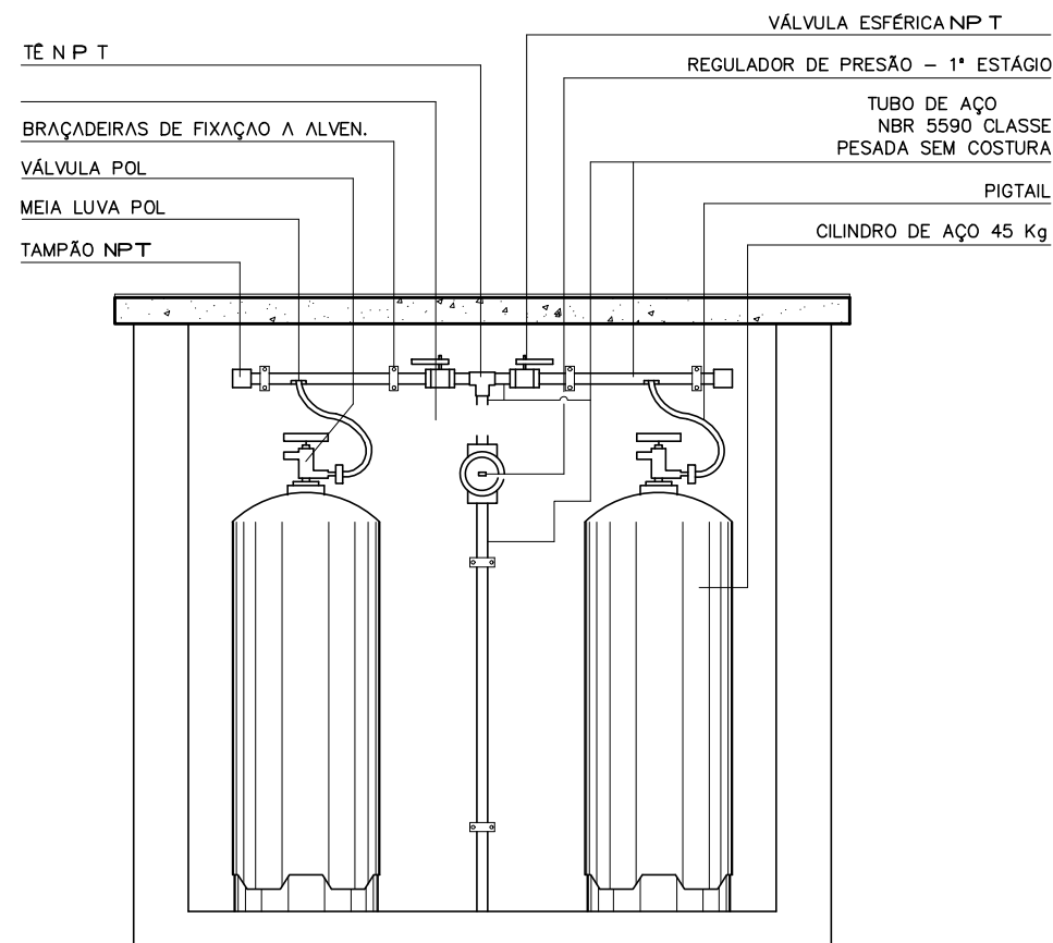
CORTE BB SEM ESCALA
