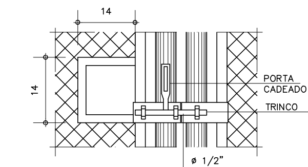
DETALHE 2 - FECHO CADEADO SEM ESCALA
