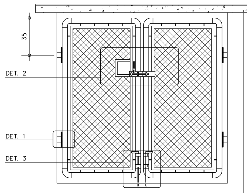
VISTA A SEM ESCALA
