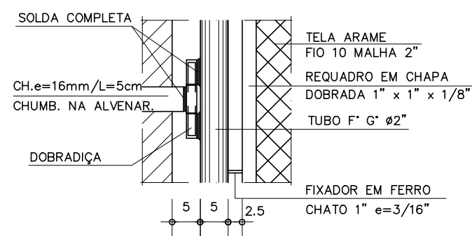
DETALHE 1 - DOBRADIÇA SEM ESCALA
