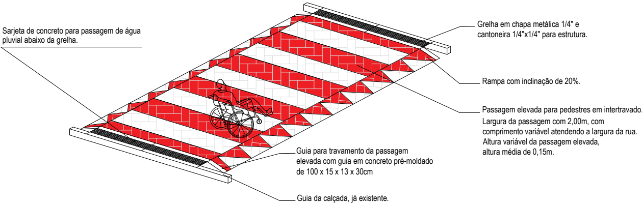
DETALHE DA PASSAGEM ELEVADA. sem escala
