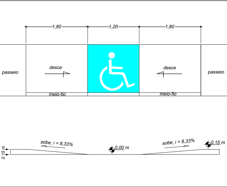
EXECUTIVO DA RAMPA. sem escala
