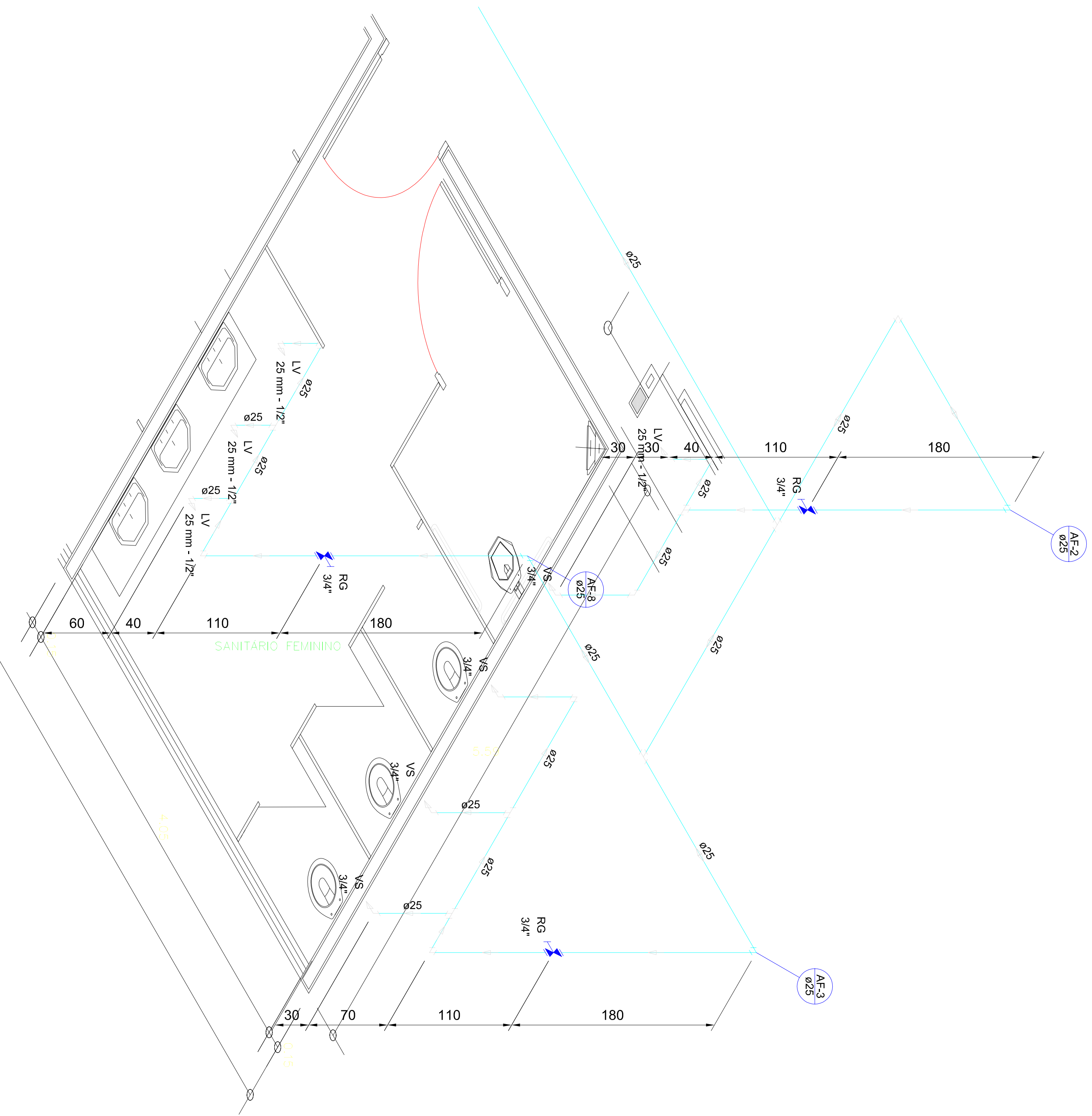
Detalhe H6 escala 1:25
