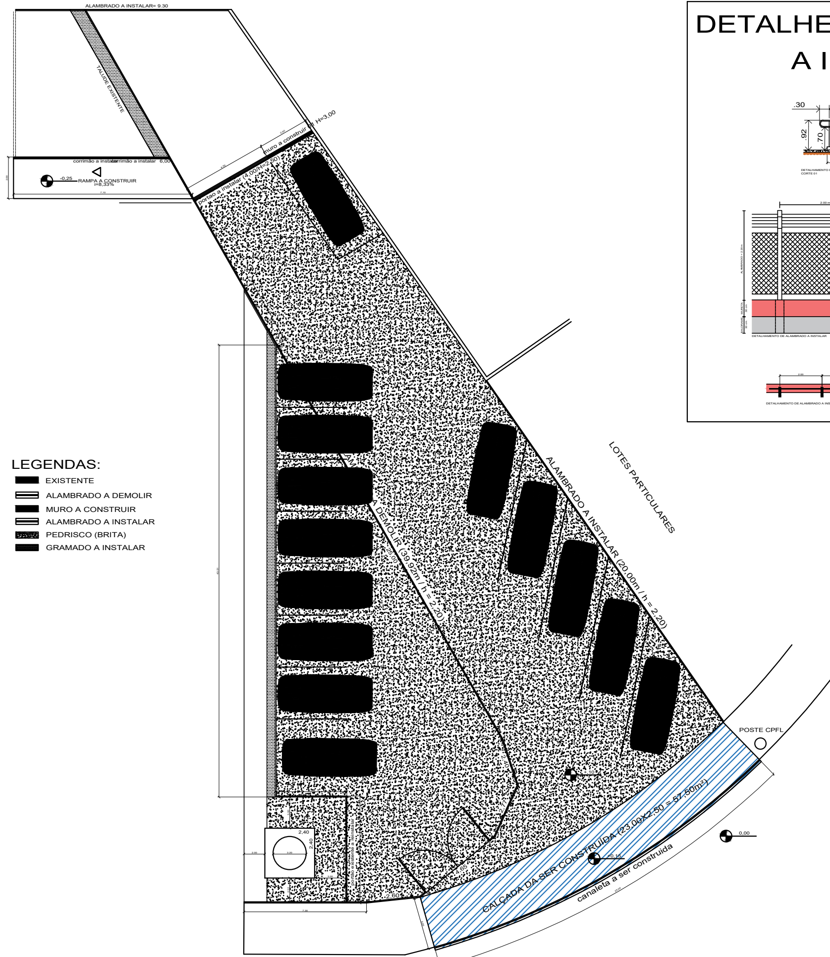
PLANTA (ESC. 1/25)
