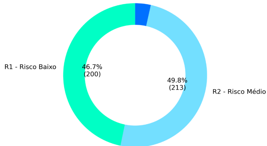
Figura 6.1-1. Porcentagem e valores absolutos de risco e vulnerabilidade a processos hidrológicos do município de Pindamonhangaba.
