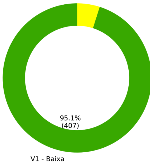
Figura 6.1-1. Porcentagem e valores absolutos de risco e vulnerabilidade a processos hidrológicos do município de Pindamonhangaba.
