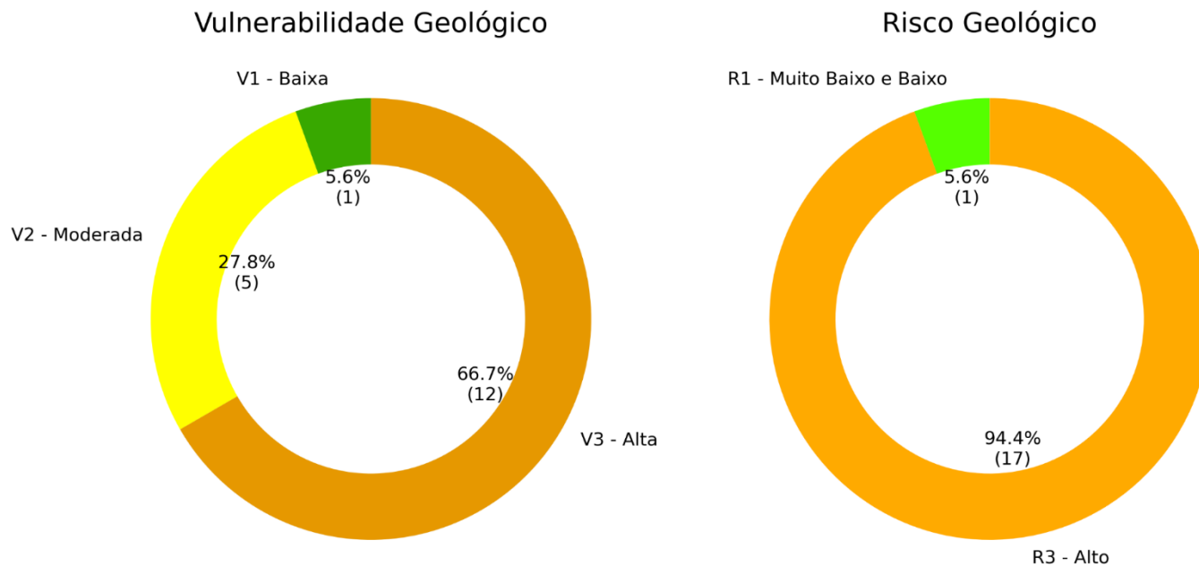
Figura 5.1-1. Porcentagem e valores absolutos de risco e vulnerabilidade a processos geológicos do município de Pindamonhangaba.
