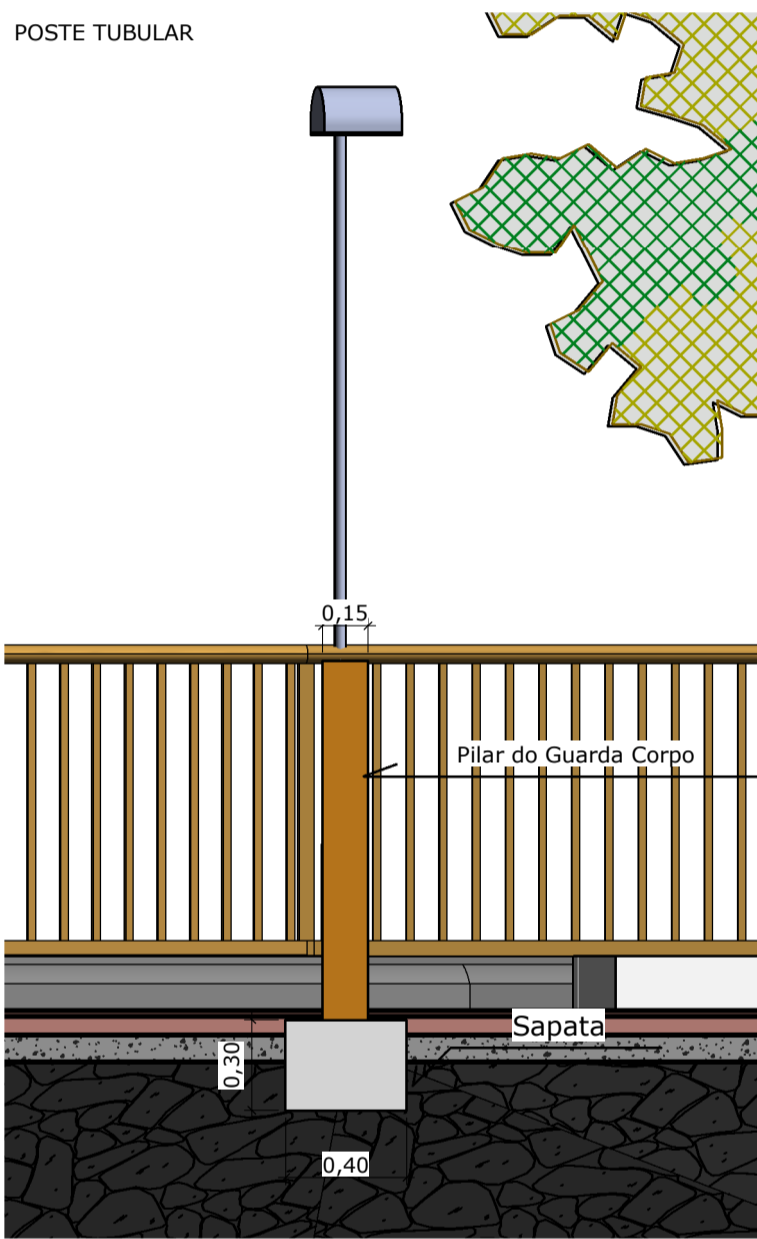
5 Det. Pilar Guarda corpo 1 : 25
