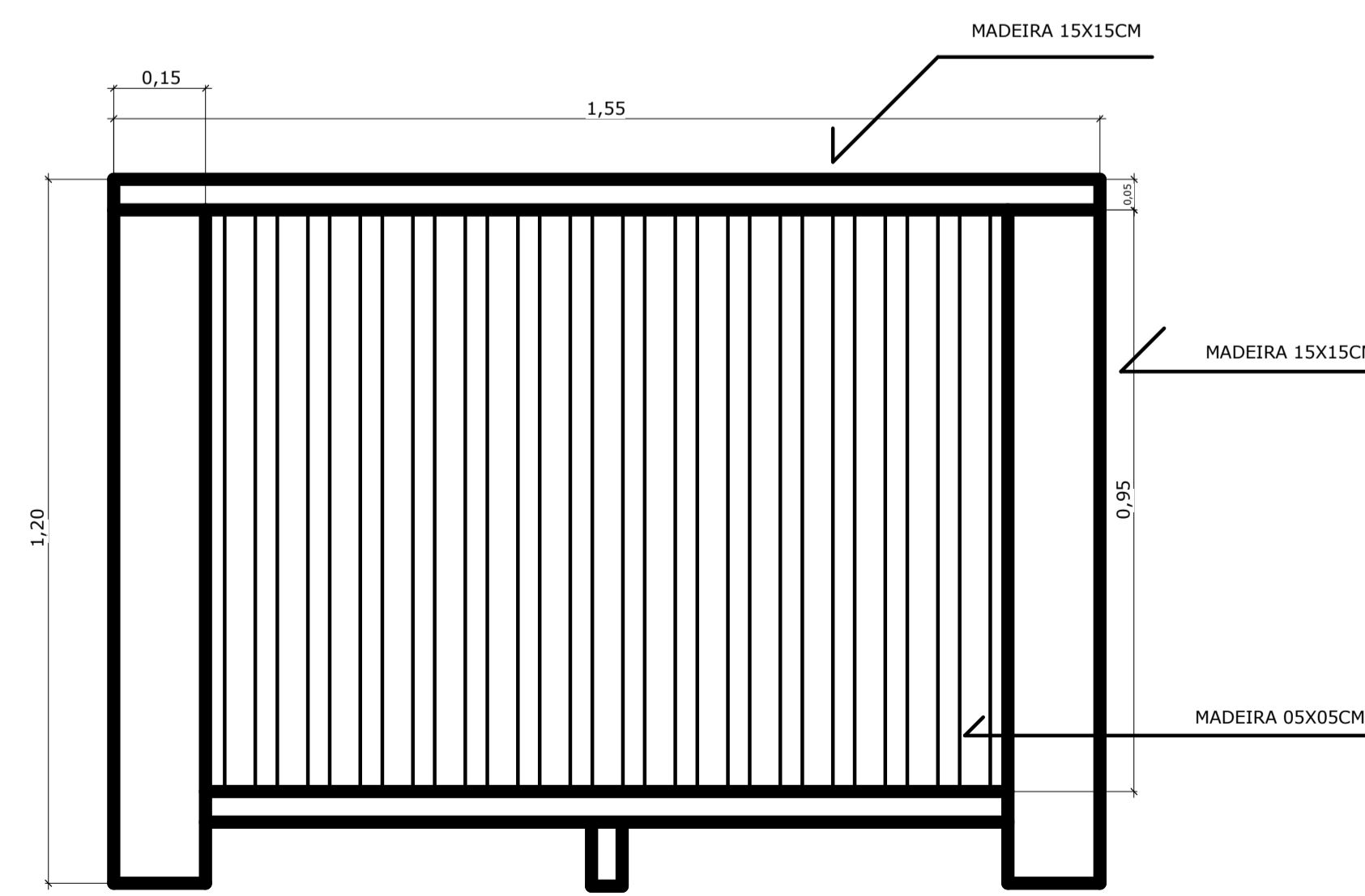
2 Det. Guarda Corpo Madeira Sem escala
