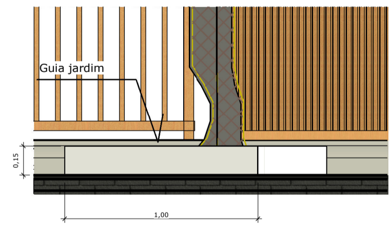
3 Det. Jardineira 1 : 20
