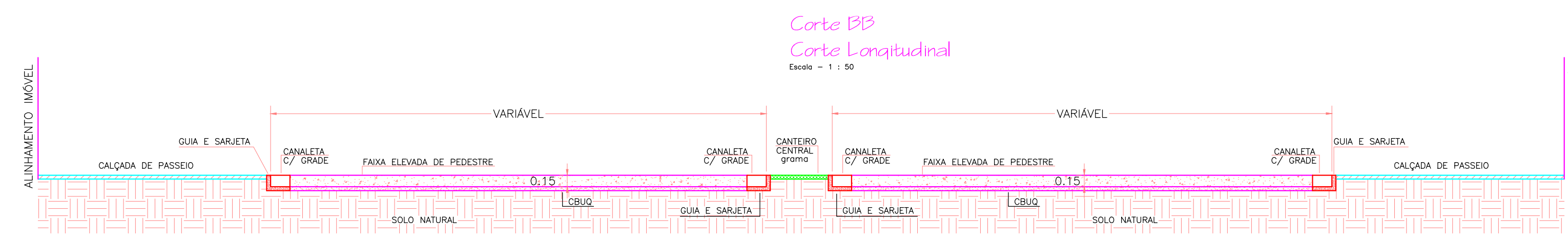
Avenida Rui Barbosa Rampa de Acesso e Faixa Elevada de Pedestres Rebassamento de calçada sem rampas complementares Data: 11/20
