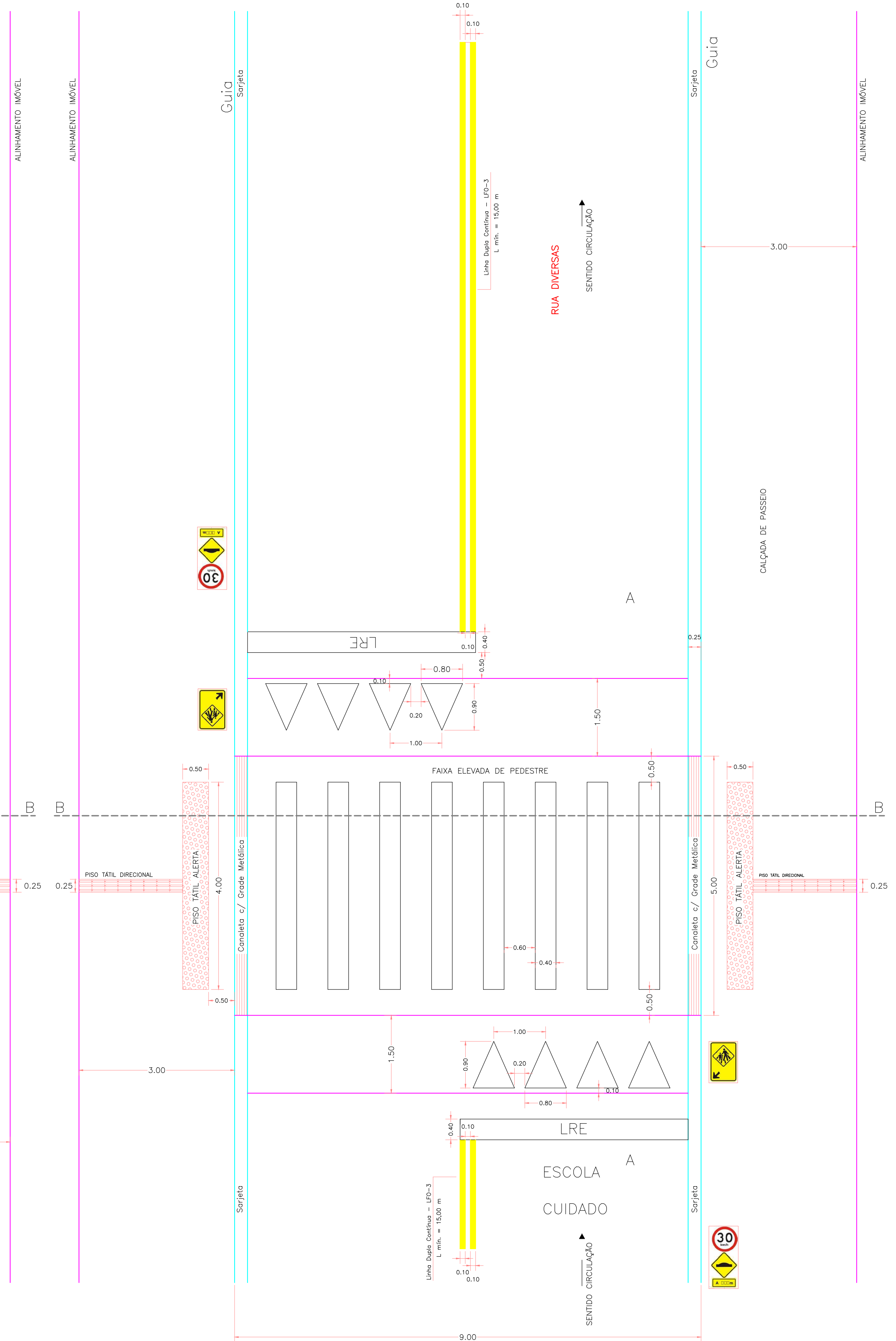
RUA DE SENTIDO DUPLO DE TRÁFEGO Rampa de Acesso e Faixa Elevada de Pedestres Rebassamento de calçada sem rampas complementares Data: 11/20
