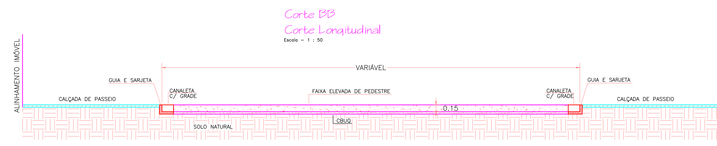
RUA DE SENTIDO DUPLO DE TRÁFEGO Rampa de Acesso e Faixa Elevada de Pedestres Rebassamento de calçada sem rampas complementares Data: 11/20
