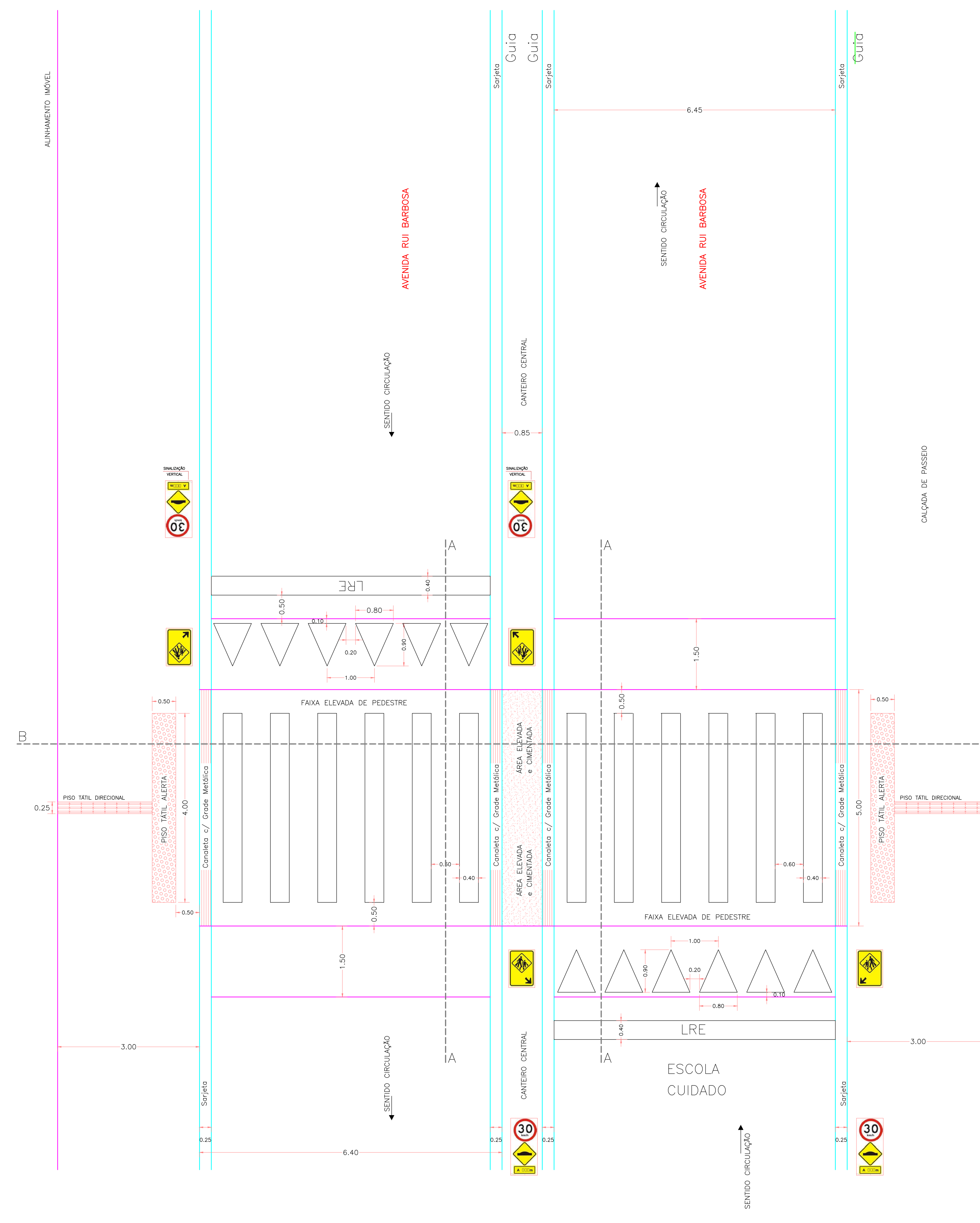
Avenida Rui Barbosa Rampa de Acesso e Faixa Elevada de Pedestres Rebassamento de calçada sem rampas complementares Data: 11/20
