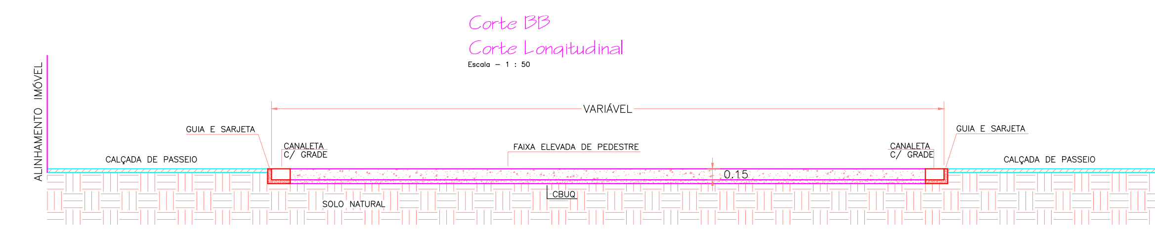
RUA DE SENTIDO ÚNICO DE TRÁFEGO Rampa de Acesso e Faixa Elevada de Pedestres Rebassamento de calçada sem rampas complementares Data: 11/20
