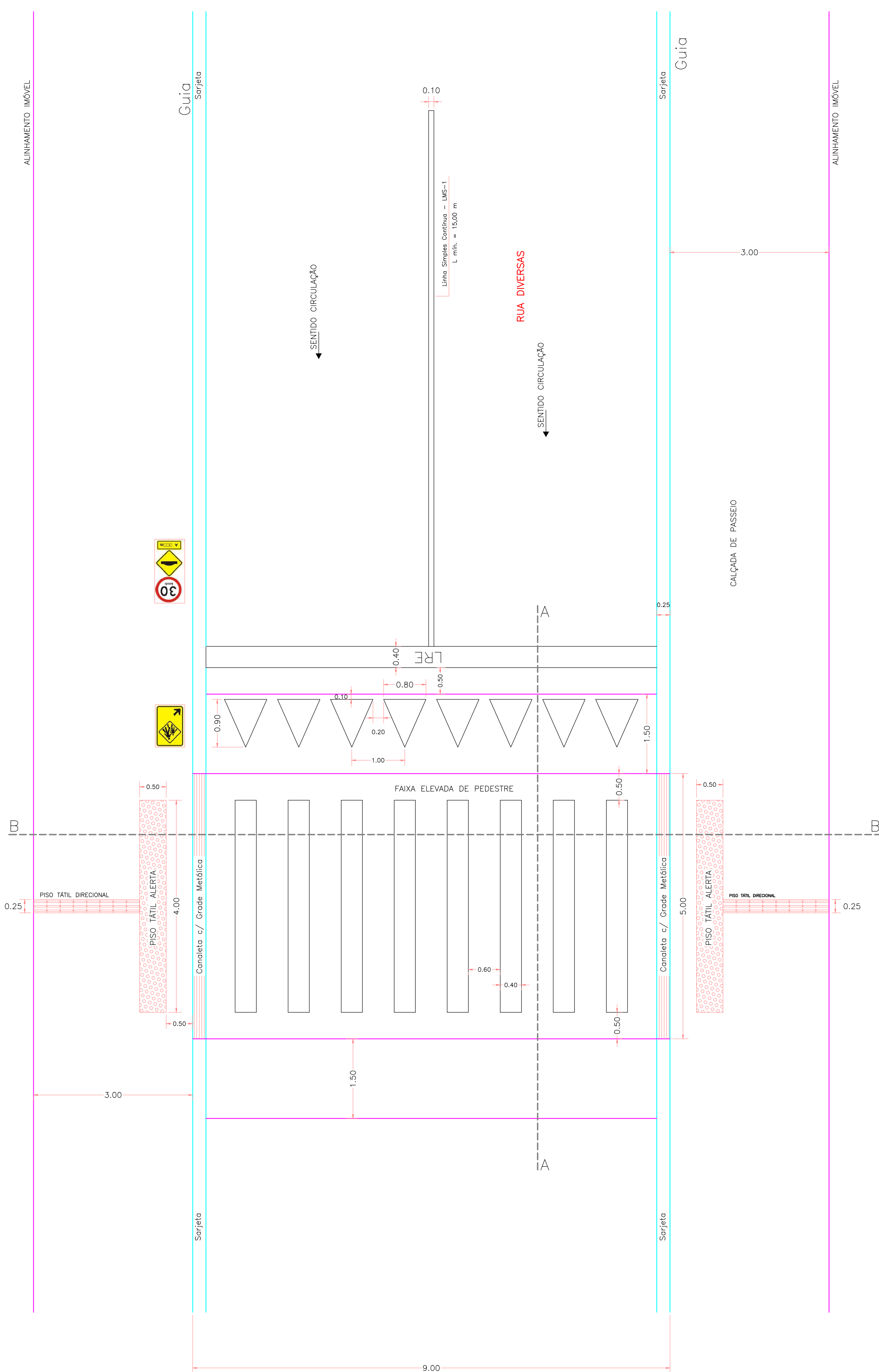
RUA DE SENTIDO ÚNICO DE TRÁFEGO Rampa de Acesso e Faixa Elevada de Pedestres Rebassamento de calçada sem rampas complementares Data: 11/20
