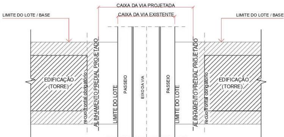
PLANTA DE FACHADA ATIVA NO ALINHAMENTO PREDIAL PROJETADO S/ ESCALA
