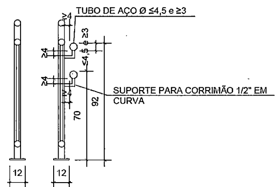
DETALHE GUARDA CORPO / CORRIMÃO
