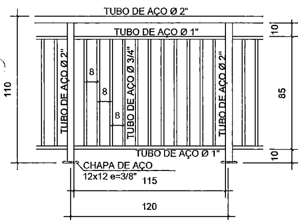
DETALHE GUARDA CORPO
