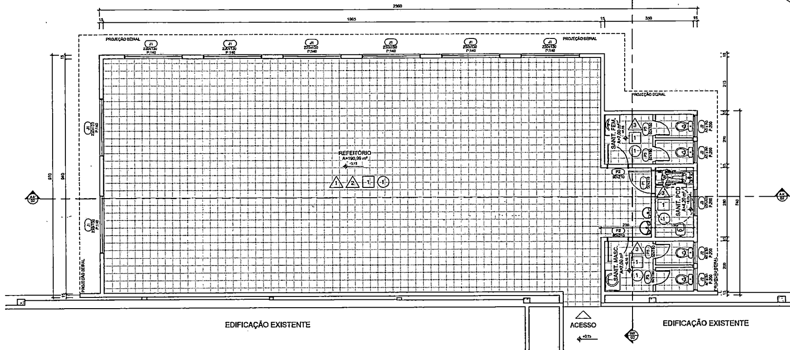
1 PLANTA BAIXA 1:50 ÁREA TOTAL CONSTRUÍDA: 221,36 m²
