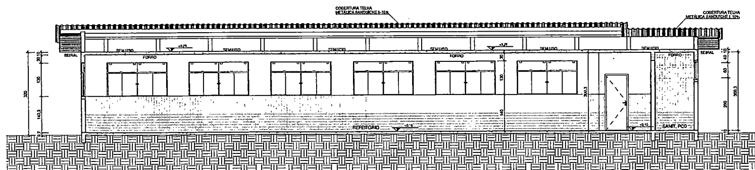
AA CORTE AA' 1:50
