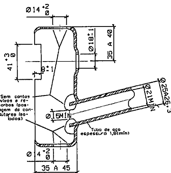
CORTE AB
