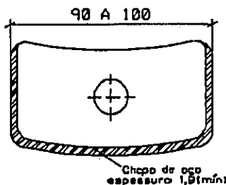
CORTE CD
