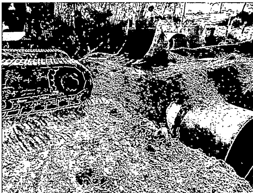
Figura 7 - Tubulação danificada substituída por tubo de 1200mm e aterrada com bica corrida
