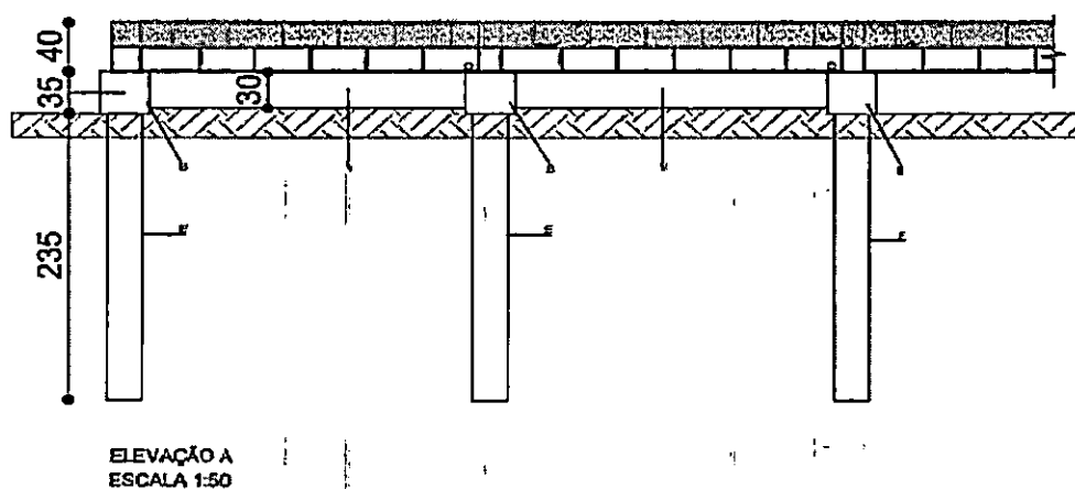
Figura 9 - Elevação A
