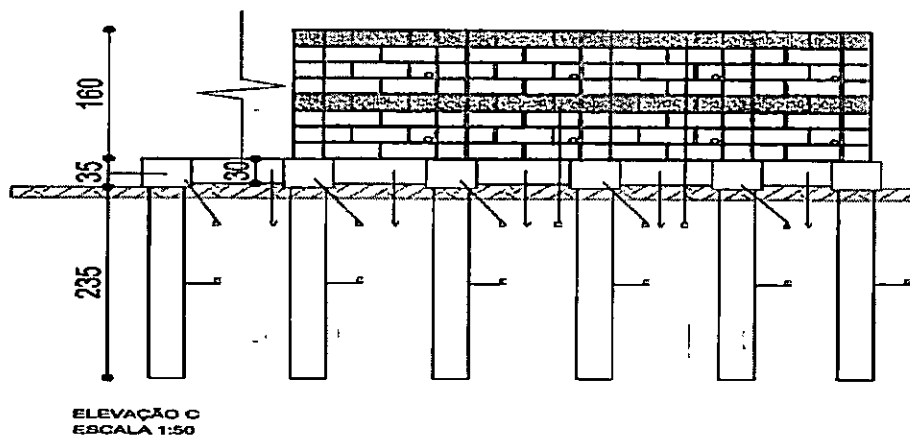
Figura 11 - Elevação C
