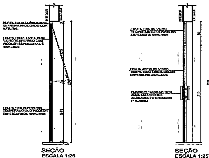
Figura 23 - Seção
