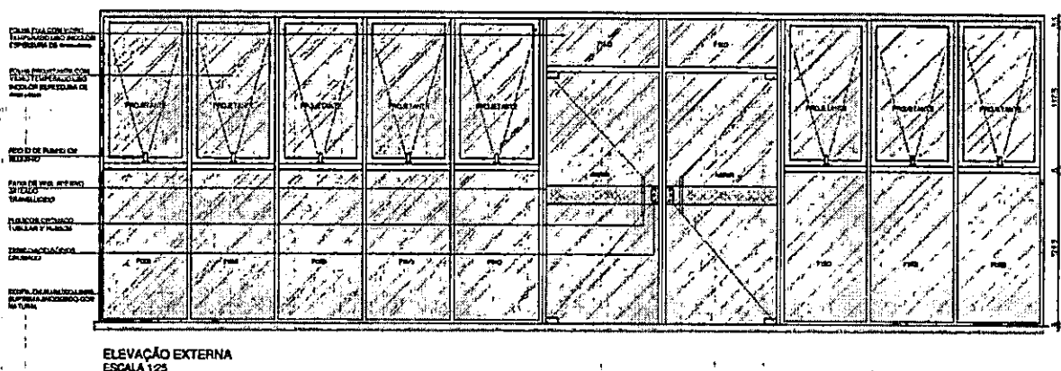
Figura 22 - Elevação externa – Conjunto de vidro da fachada
