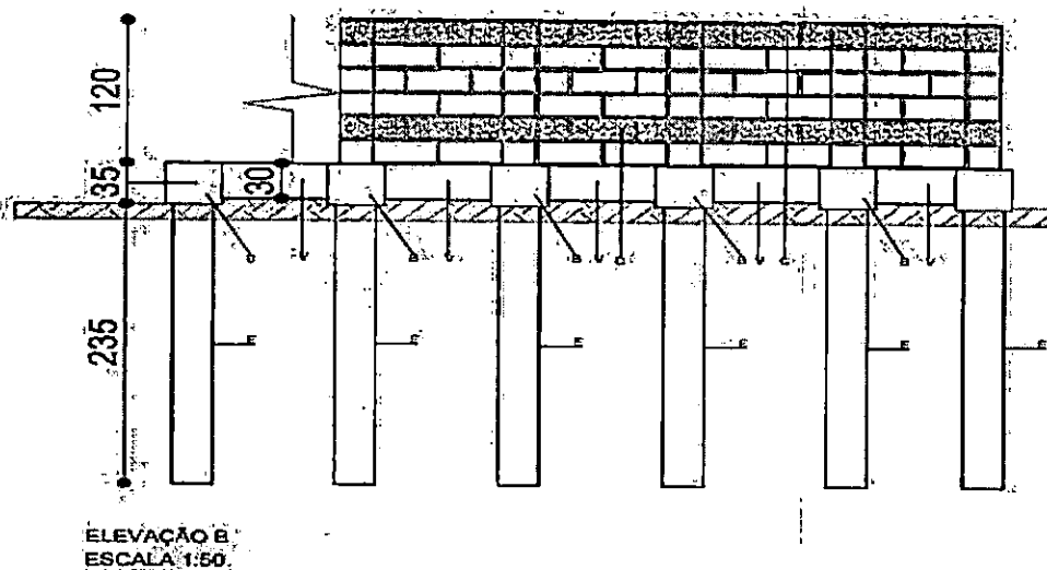
Figura 10 - Elevação B
