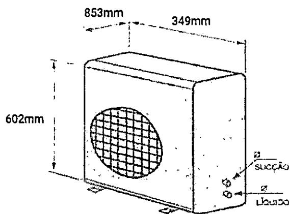
UNIDADE EXTERNA (CONDENSADORA)
