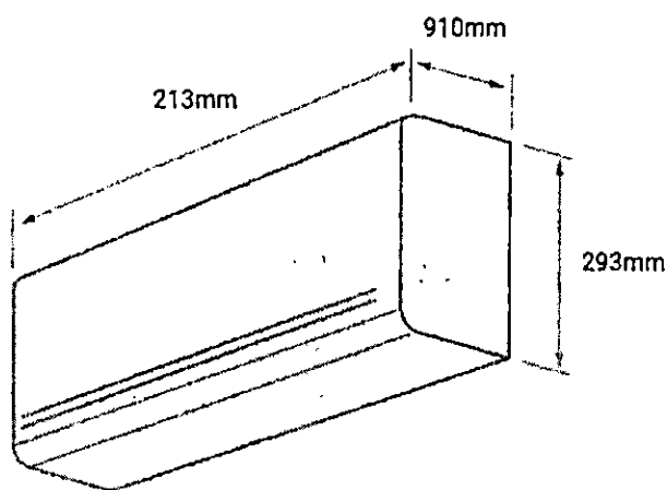
UNIDADE INTERNA (EVAPORADORA)
