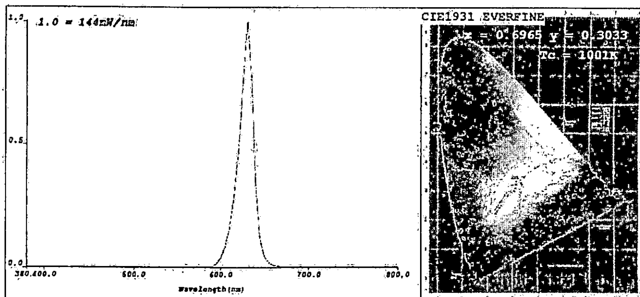
Figura 02 – Gráfico de cor – Vermelho 220 Volts
