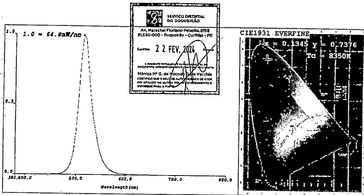
Figura 04 - Gráfico de cor - Verde 220 Volts
