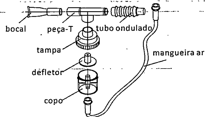
Figura 7: Componentes do nebulizador
