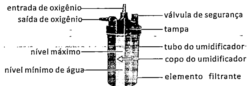
Figura 4: componentes do umidificador.
