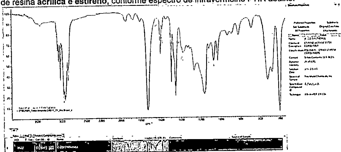
Espectrograma de infravermelho da resina da tinta
