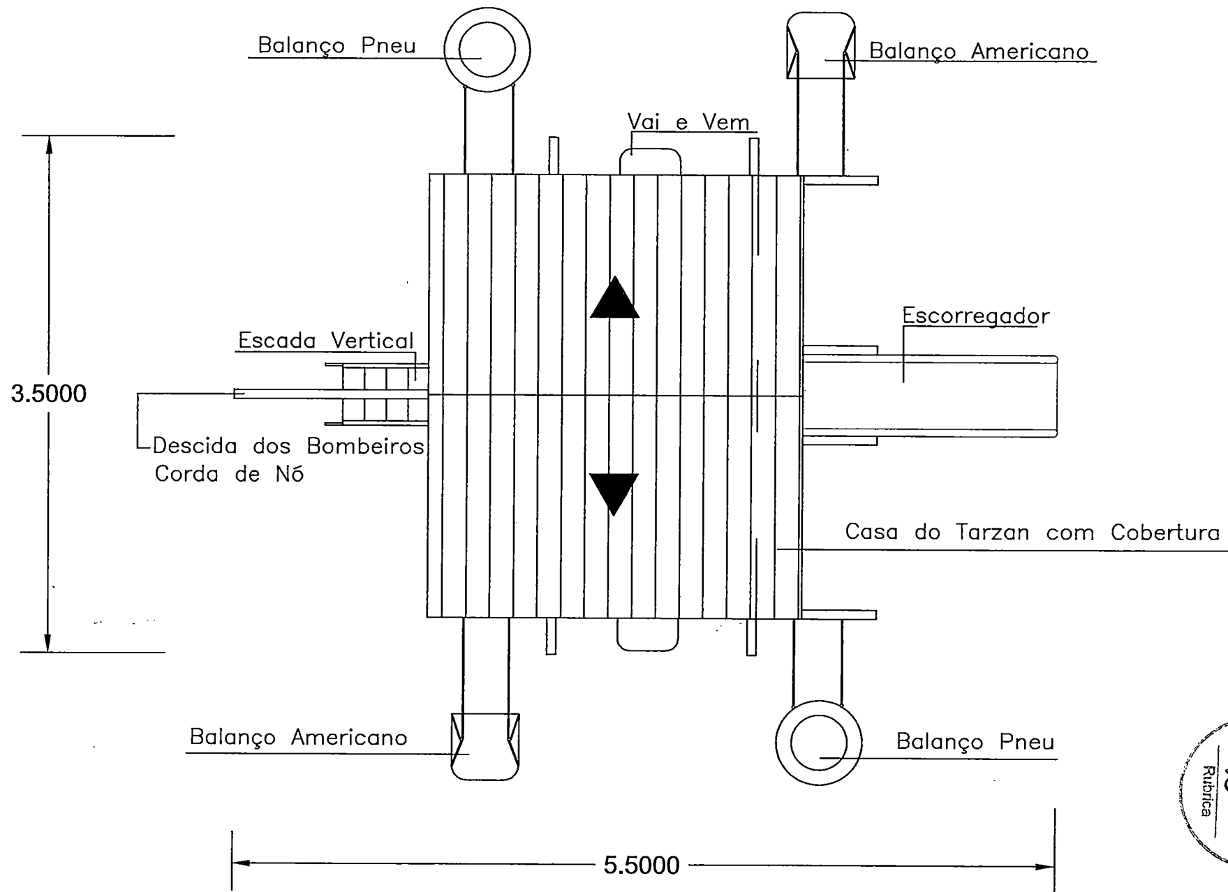
Planta Baixa Casa do Tarzan
