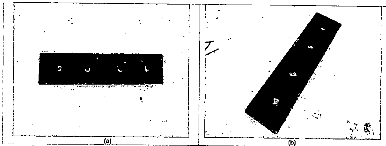
Figura 19 (a) e (b): Macrofoto evidenciando amostra após 2160 h de exposição à névoa salina.
