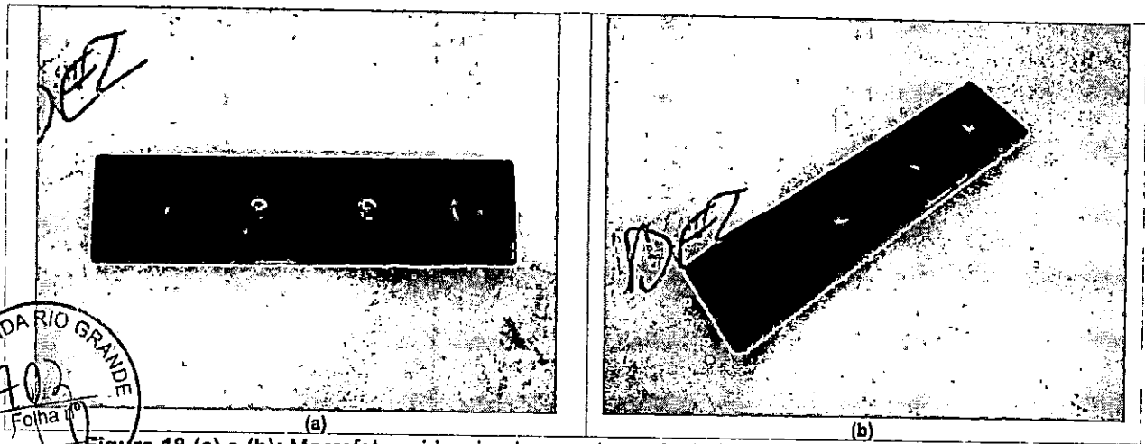
Figura 18 (a) e (b): Macrofoto evidenciando amostra após 1944 h de exposição à névoa salina.
