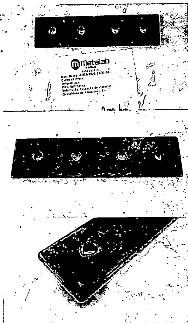
Figura 1 – Macrofotos evidenciando a amostra recebida para análise.
