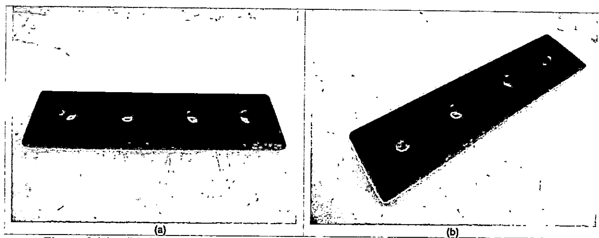
Figura 3 (a) e (b): Macrofoto evidenciando amostra após 288 h de exposição à névoa salina.
