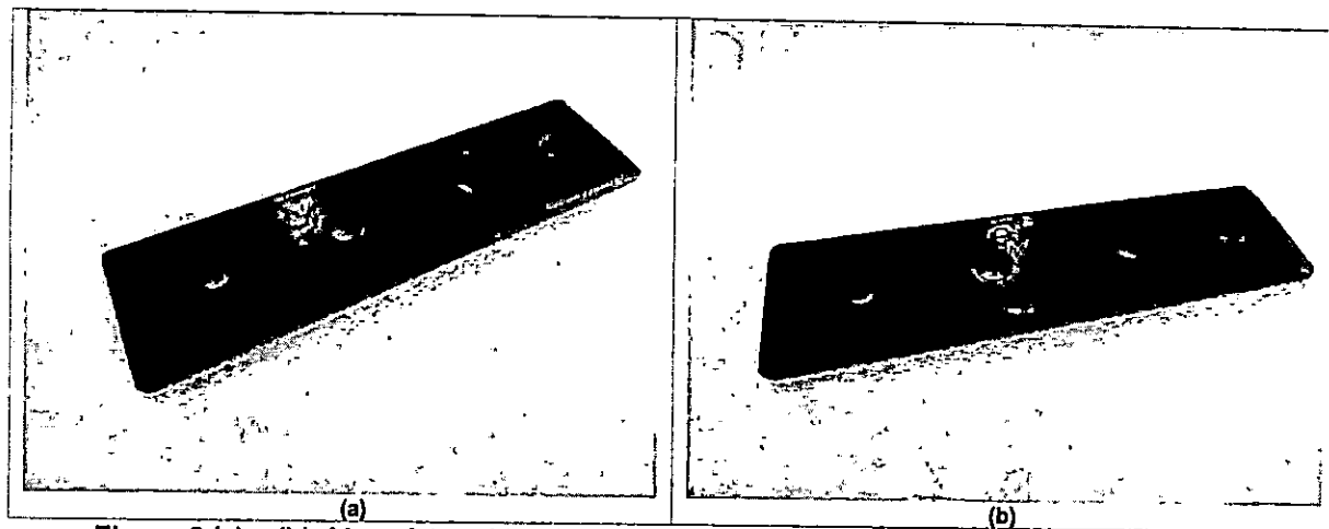
Figura 6 (a) e (b): Macrofoto evidenciando amostra após 504 h de exposição à névoa salina.
