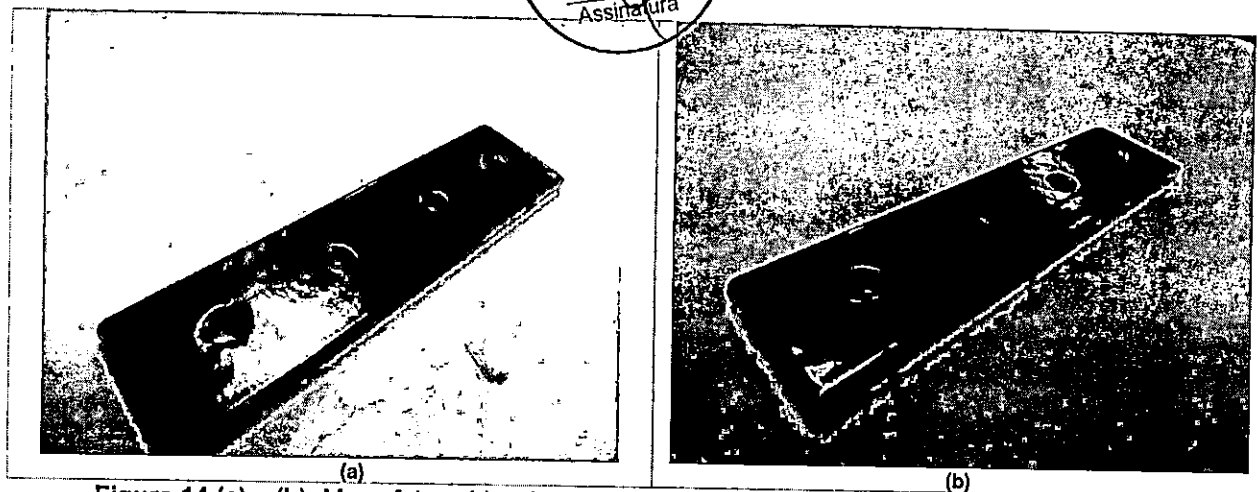
Figura 14 (a) e (b): Macrofoto evidenciando amostra após 1368 h de exposição à névoa salina.
