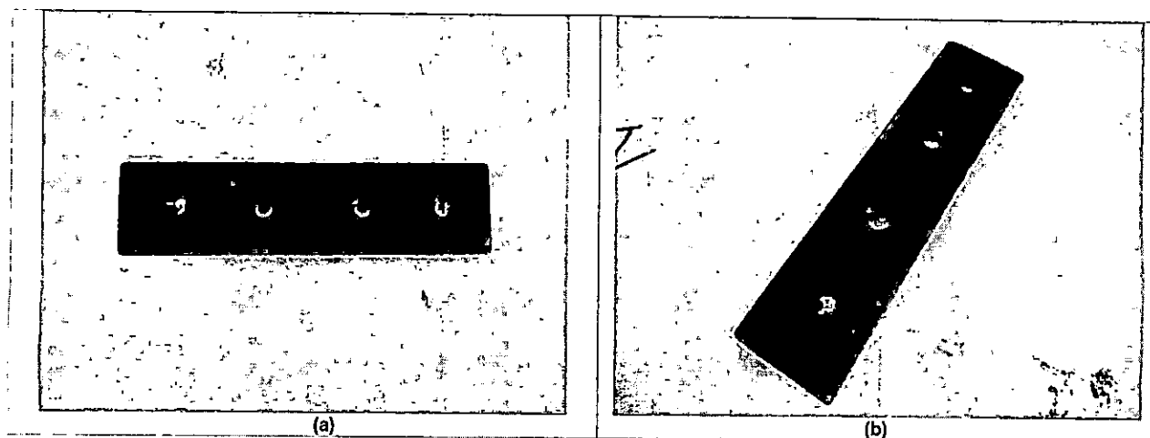
Figura 19 (a) e (b): Macrofoto evidenciando amostra após 2016 h de exposição à névoa salina.
