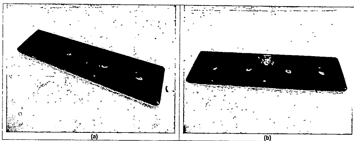
Figura 7 (a) e (b): Macrofoto evidenciando amostra após 648 h de exposição à névoa salina.
