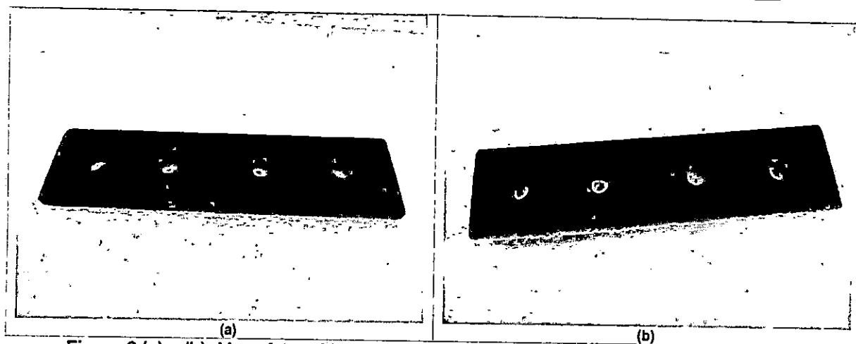
Figura 2 (a) e (b): Macrofoto evidenciando amostra após 72 h de exposição à névoa salina.
