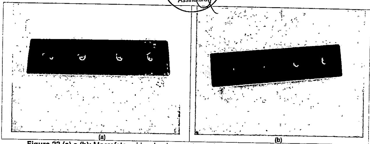
Figura 22 (a) e (b): Macrofoto evidenciando amostra após 2448 h de exposição à névoa salina.
