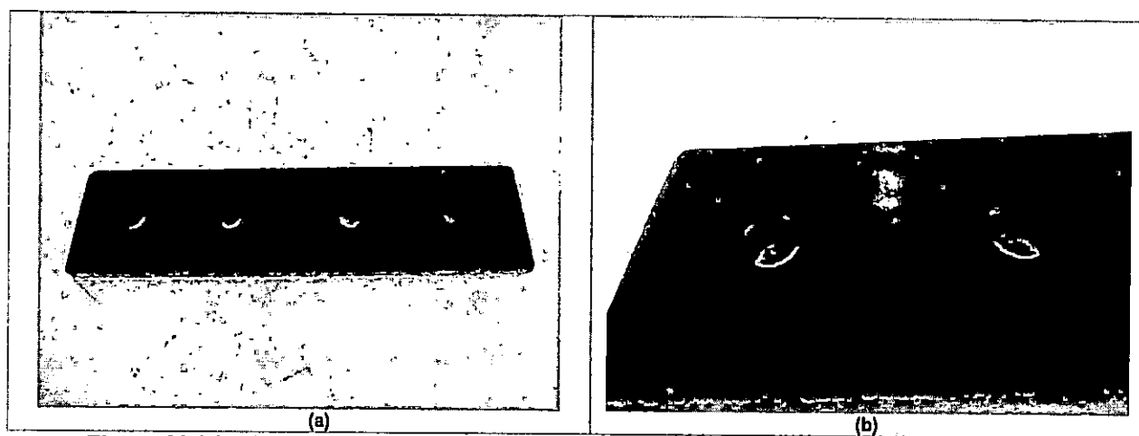
Figura 23 (a) e (b): Macrofoto evidenciando amostra após 2520 h de exposição à névoa salina.
