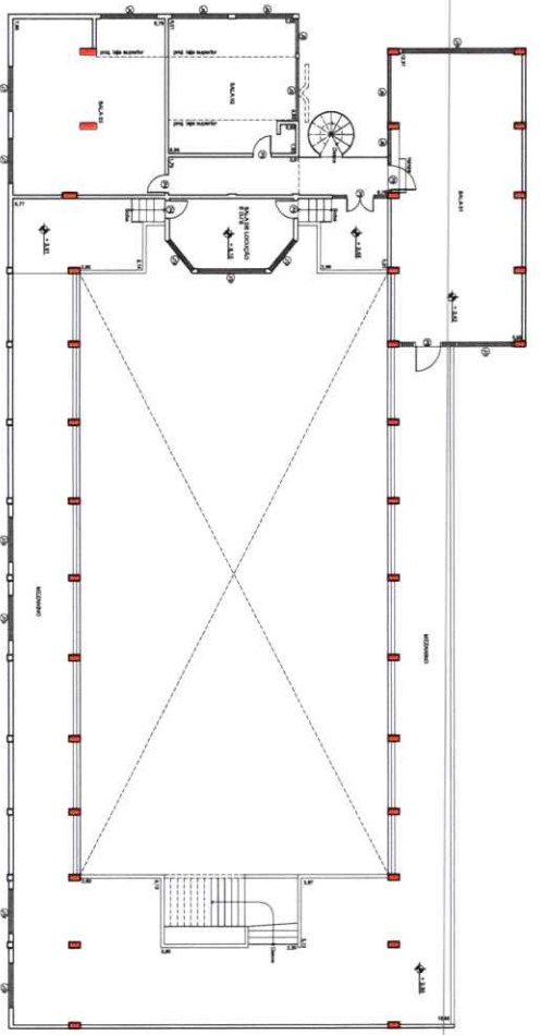
01 PLANTA BAIXA ESC: 1/25
