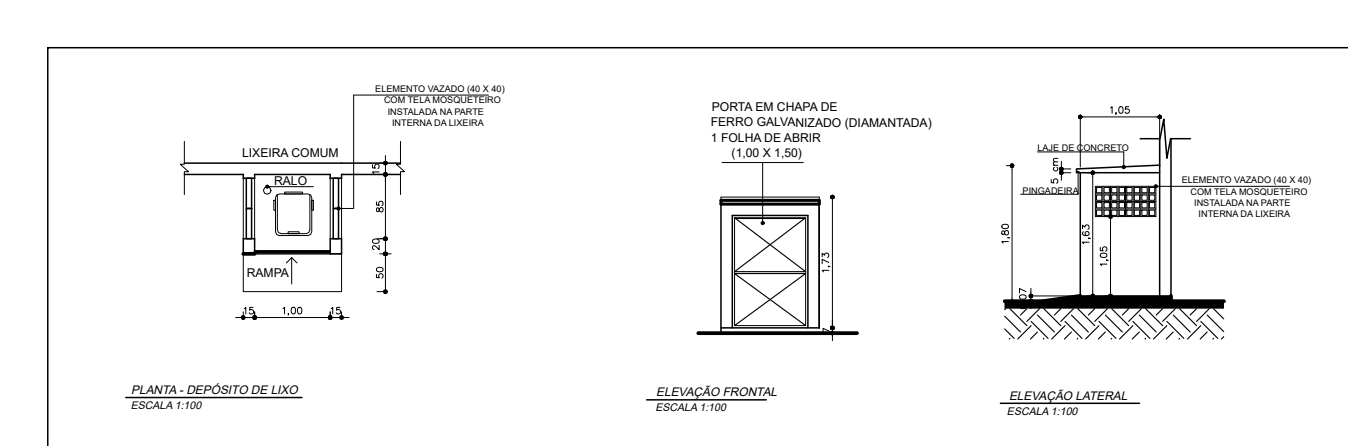
11 DET. LIXEIRA PADRÃO 1:100
