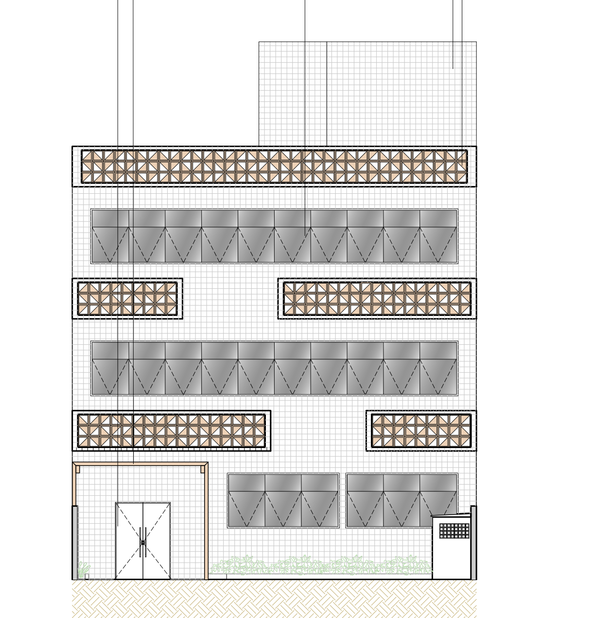
10 ELEVACÃO 01 1:100
