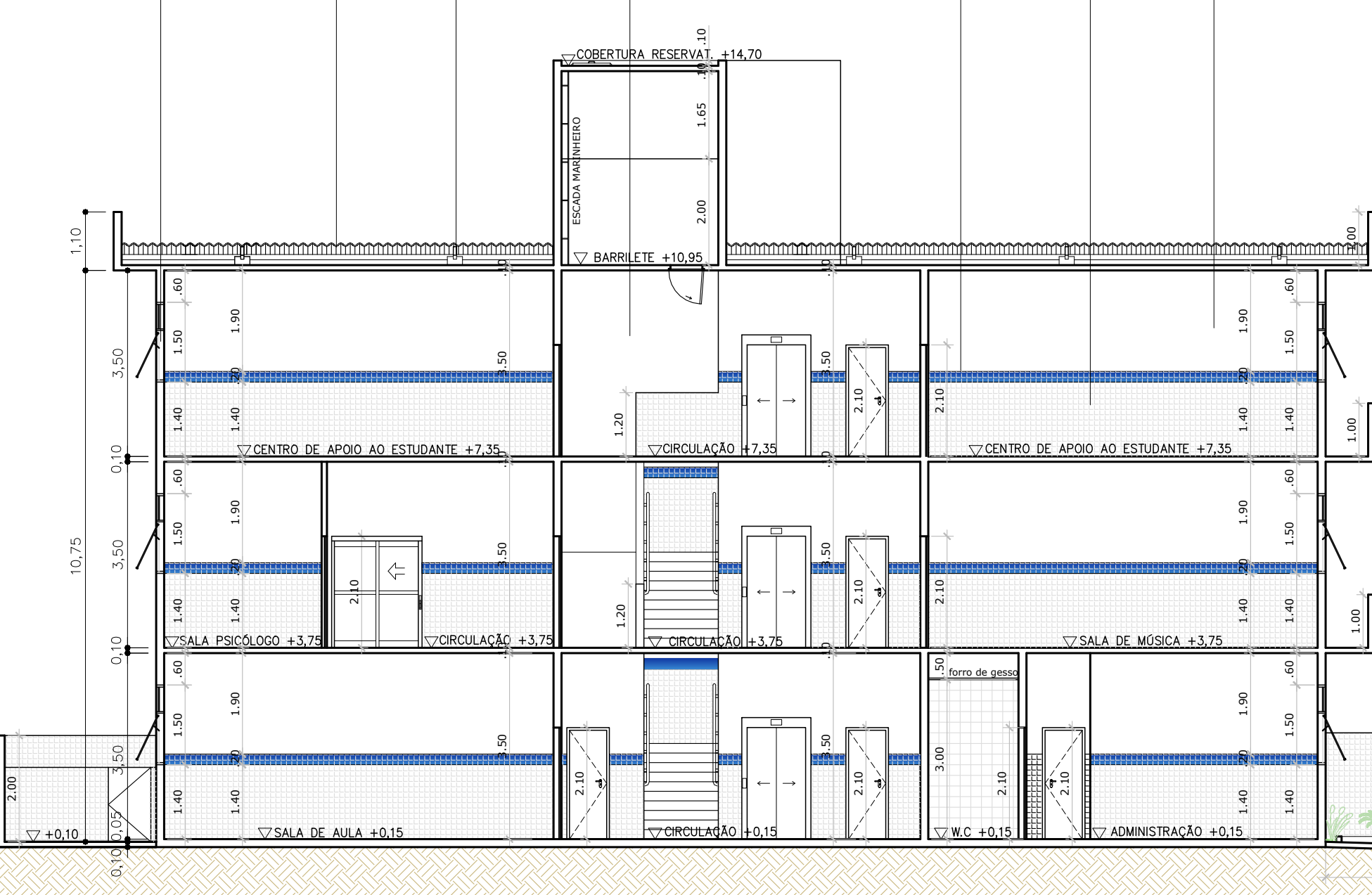
07 CORTE AA 1:100
