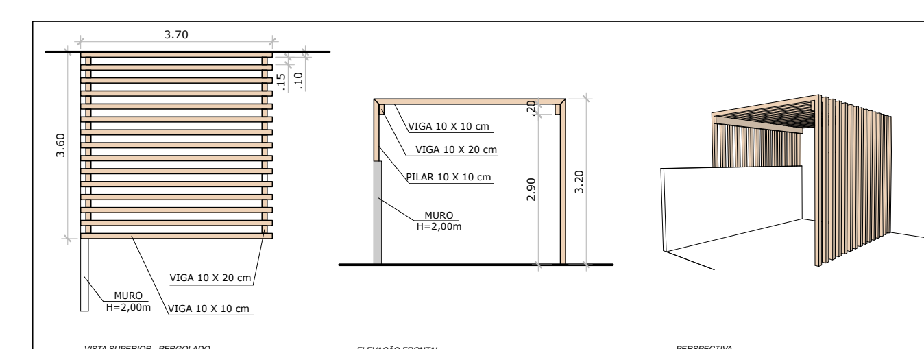
12 PERGOLADO DE MADEIRA 1:100
