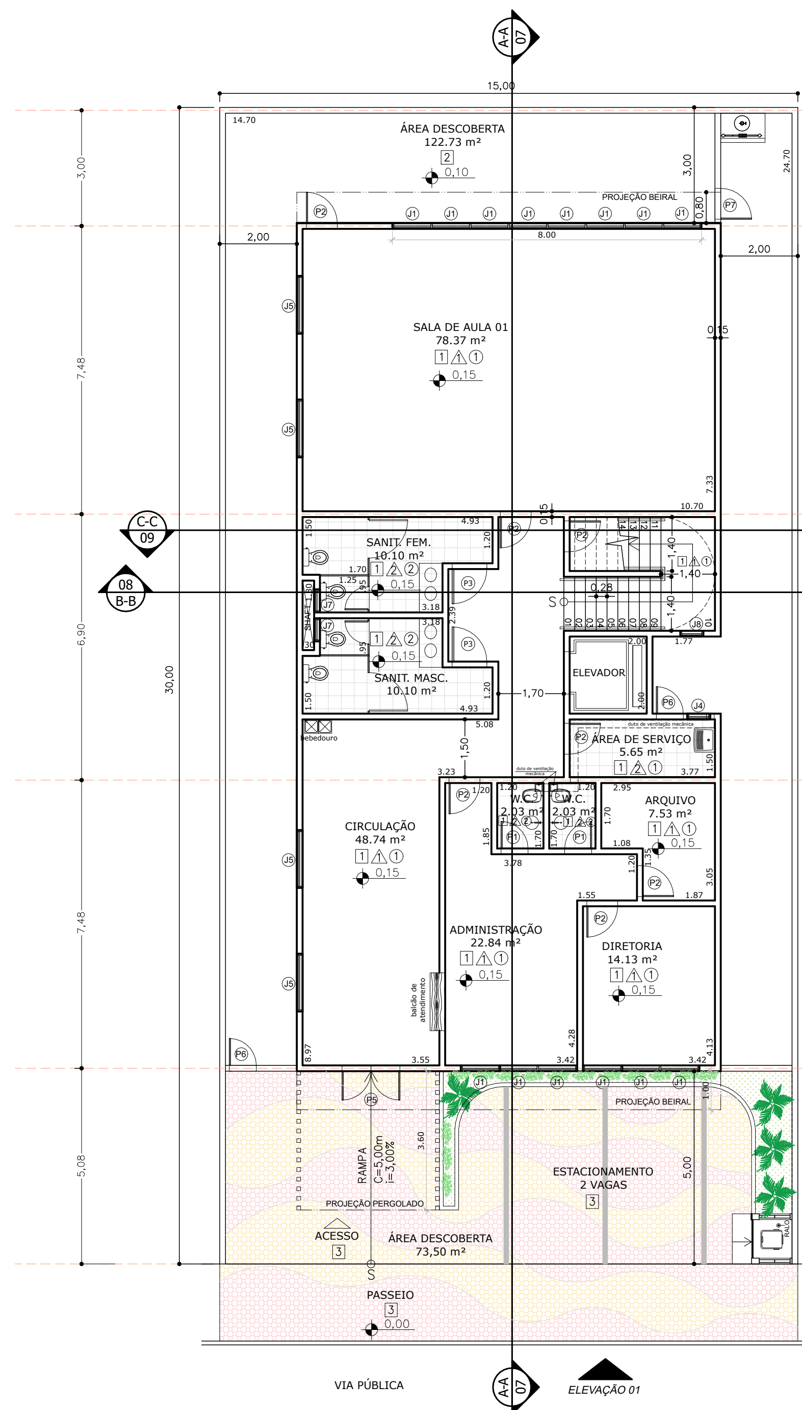
01 PLANTA TÉRREO 1:100
