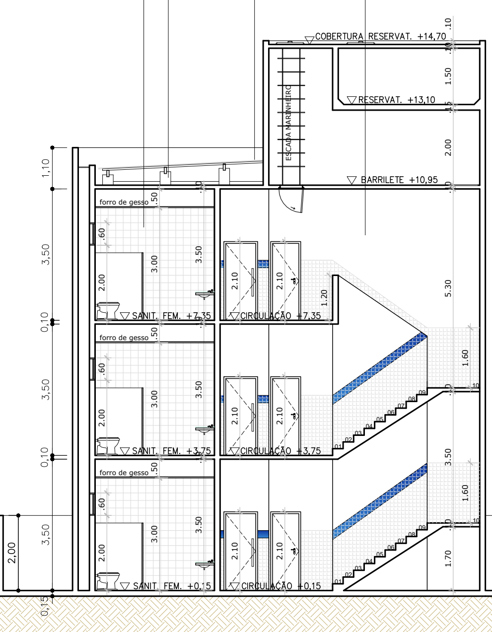
08 CORTE BB 1:100
