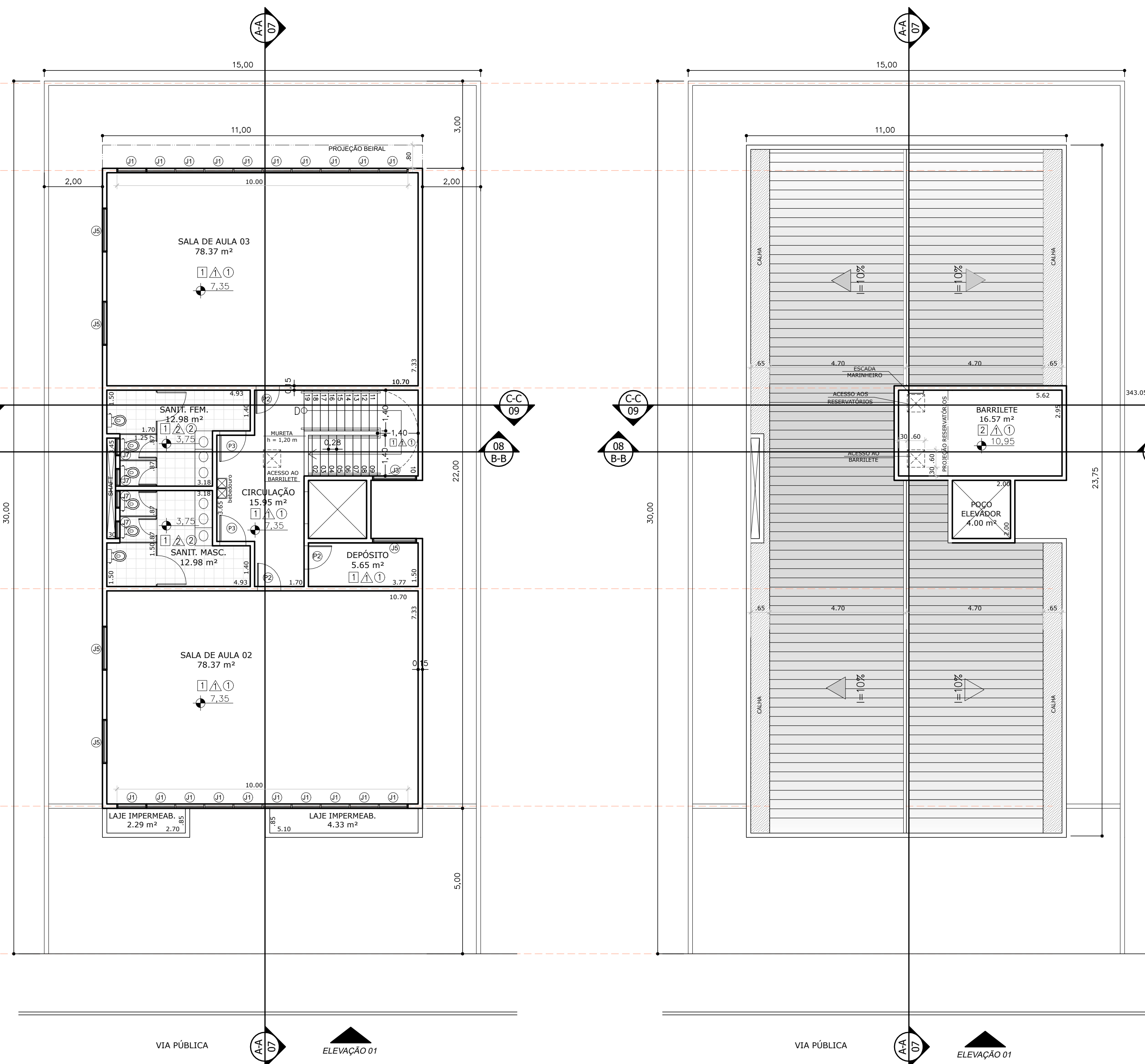
03 PLANTA 2º PAVIMENTO 1:100
