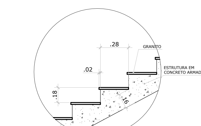
13 DET. ESCADA 1:100
