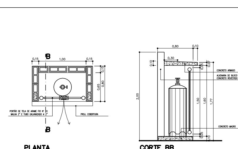
14 DET. ABRIGO DE GÁS GLP 1:100
