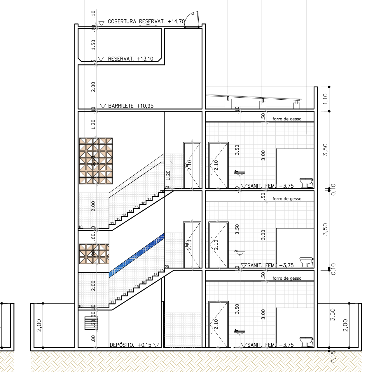
09 CORTE CC 1:100
