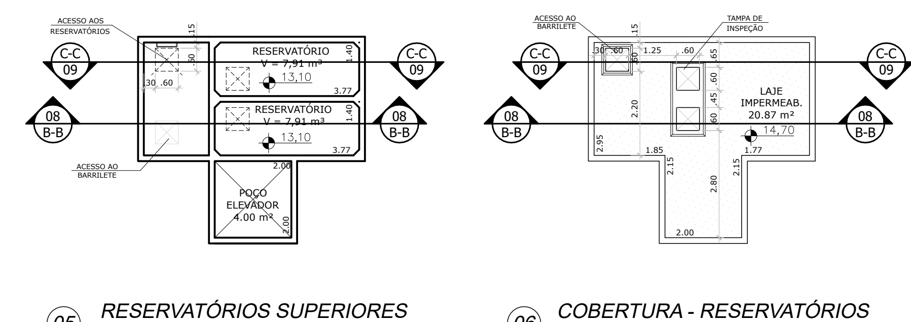
05 RESERVATÓRIOS SUPERIORES 1:100 06 COBERTURA - RESERVATÓRIOS 1:100
