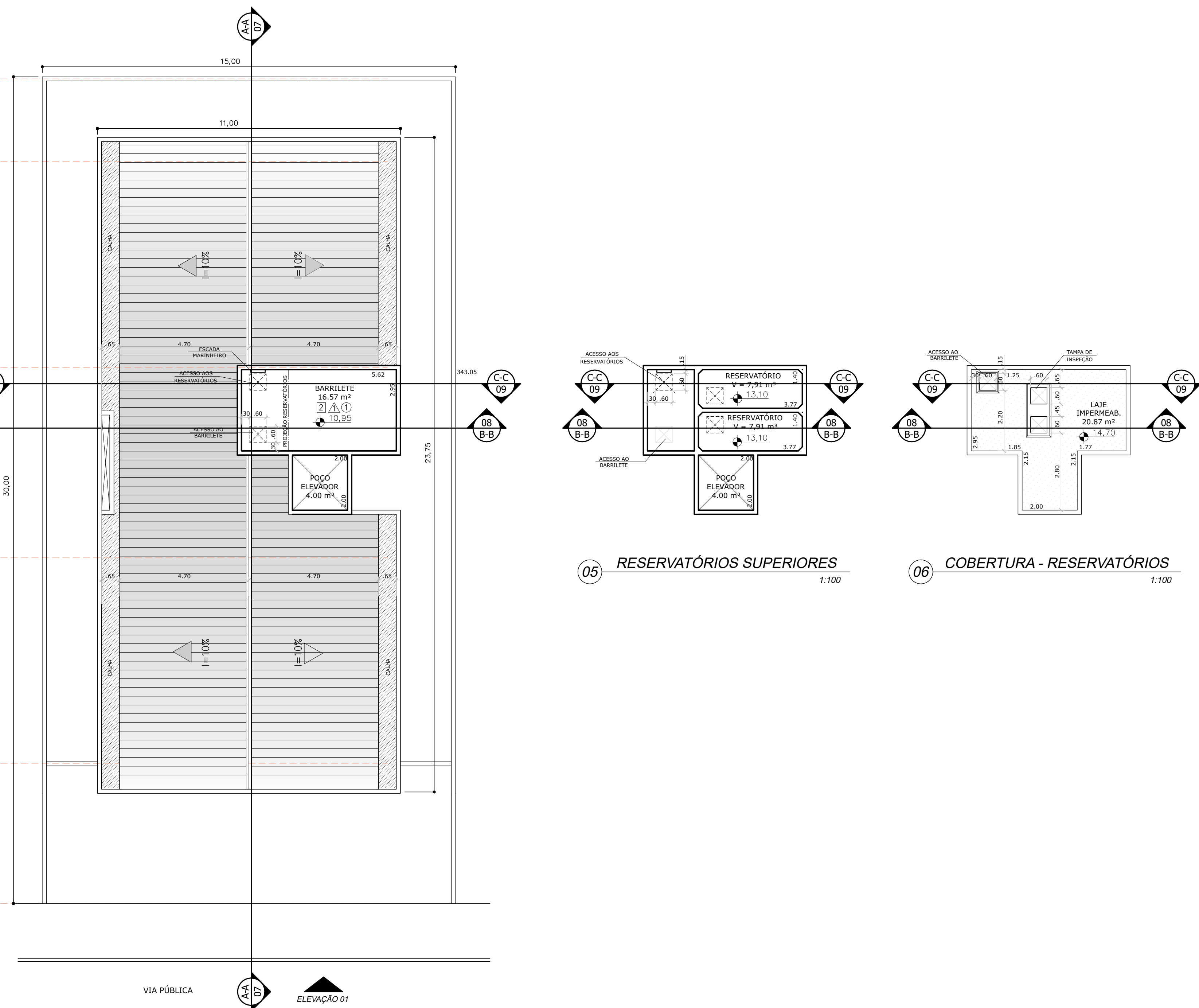
04 PLANTA COBERTURA 1:100
