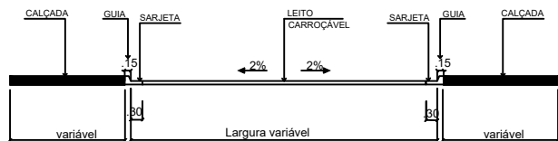
SEÇÃO TIPO - Conforme Anexos B e C Área: 4.556,78 m 2
