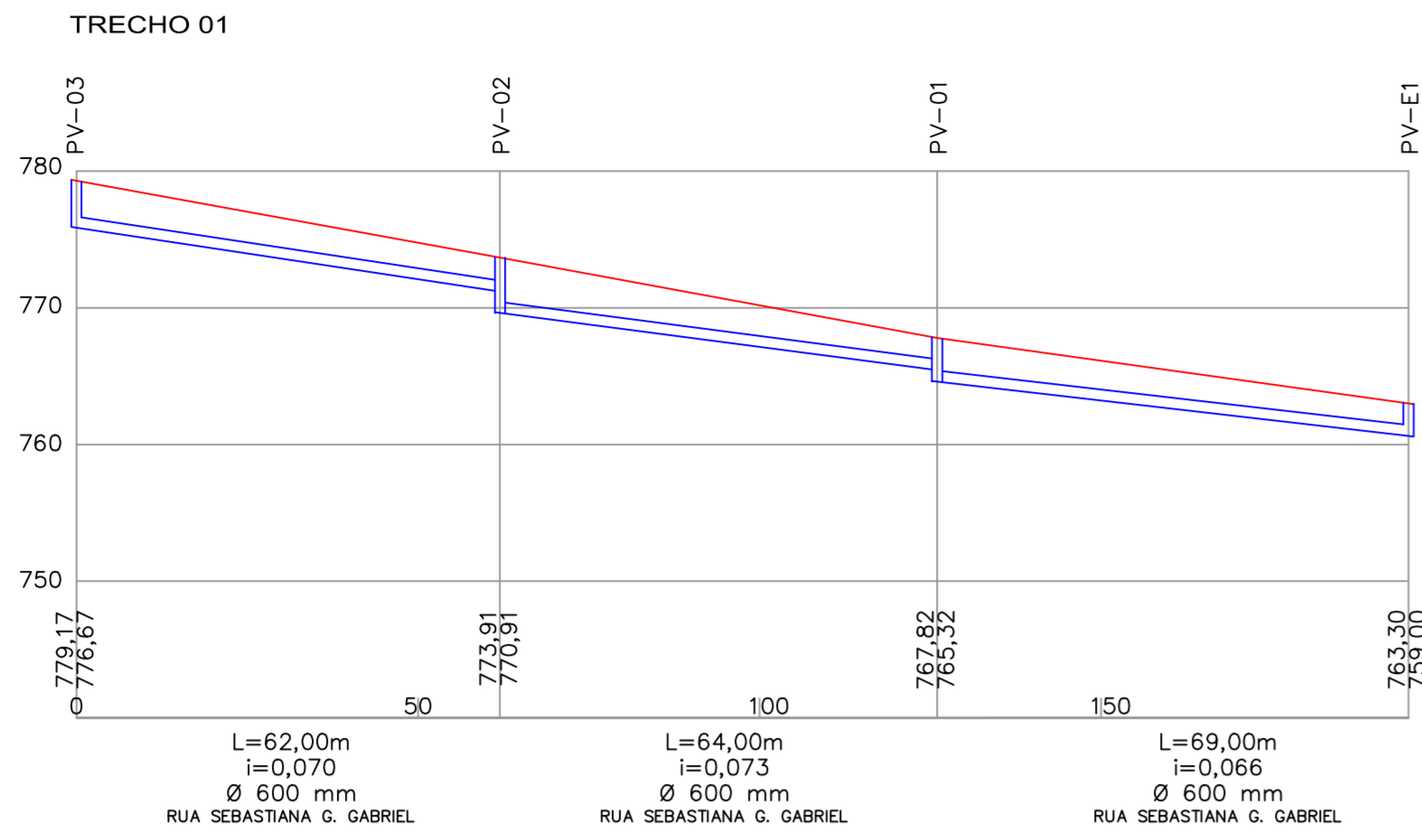
PERFIL LONGITUDINAL ESCALA H 1:100 V 1:500
