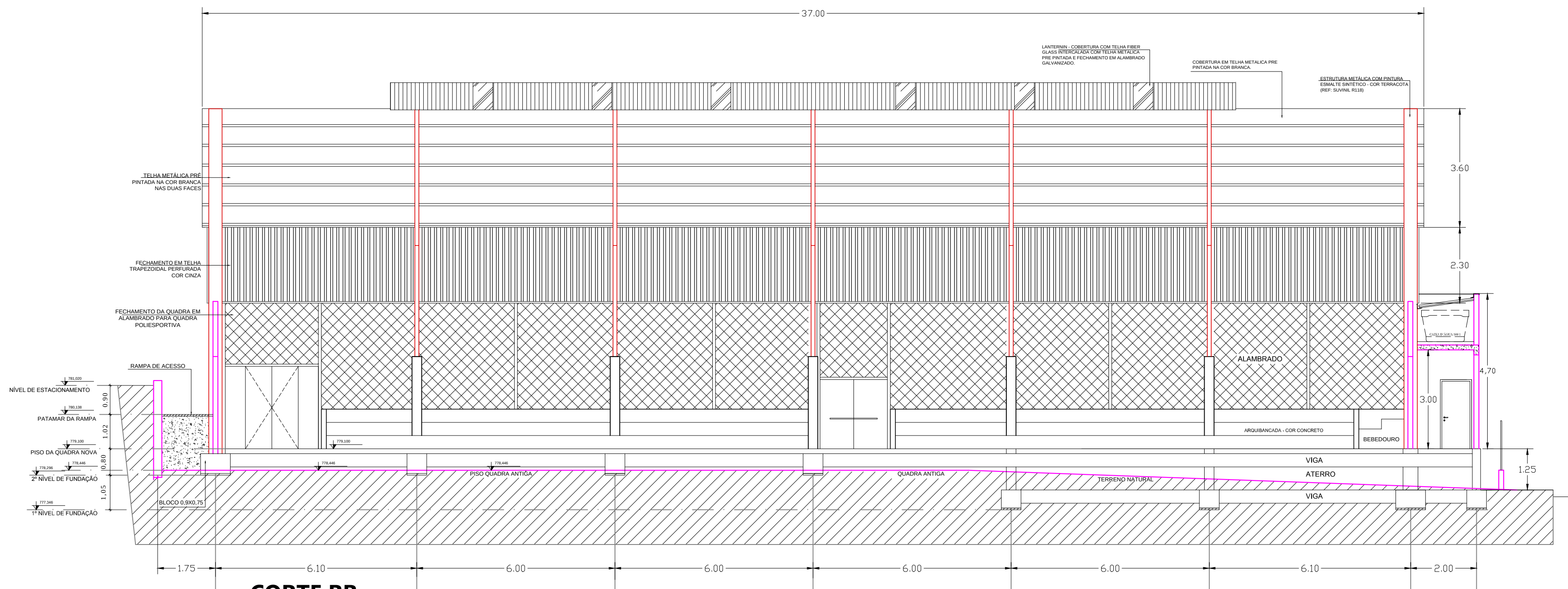
CORTE BB Esc.: 1/100
