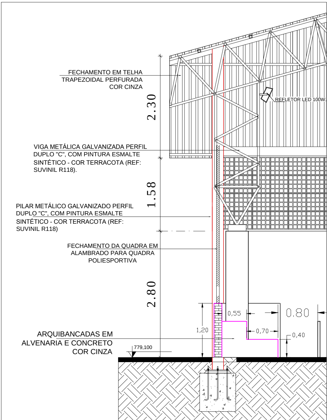
DETALHE CONSTRUTIVO Esc.: 1/50
