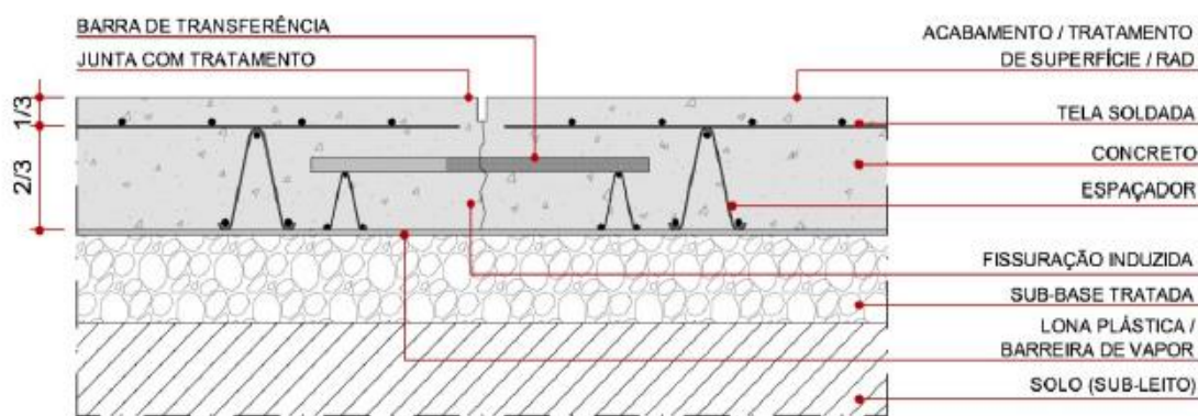
Figura 06 – Esquema de execução do piso de concreto armado polido da quadra.
