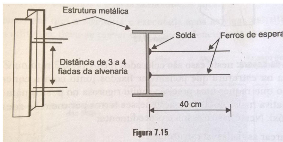
Figura 03 – Esquema de amarração entre alvenarias e pilares metálicos.
