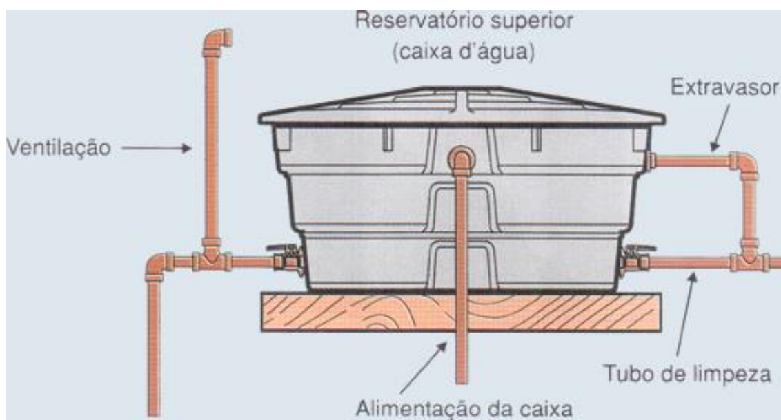
Figura 09 - Esquema de ligação das caixas d' água.
