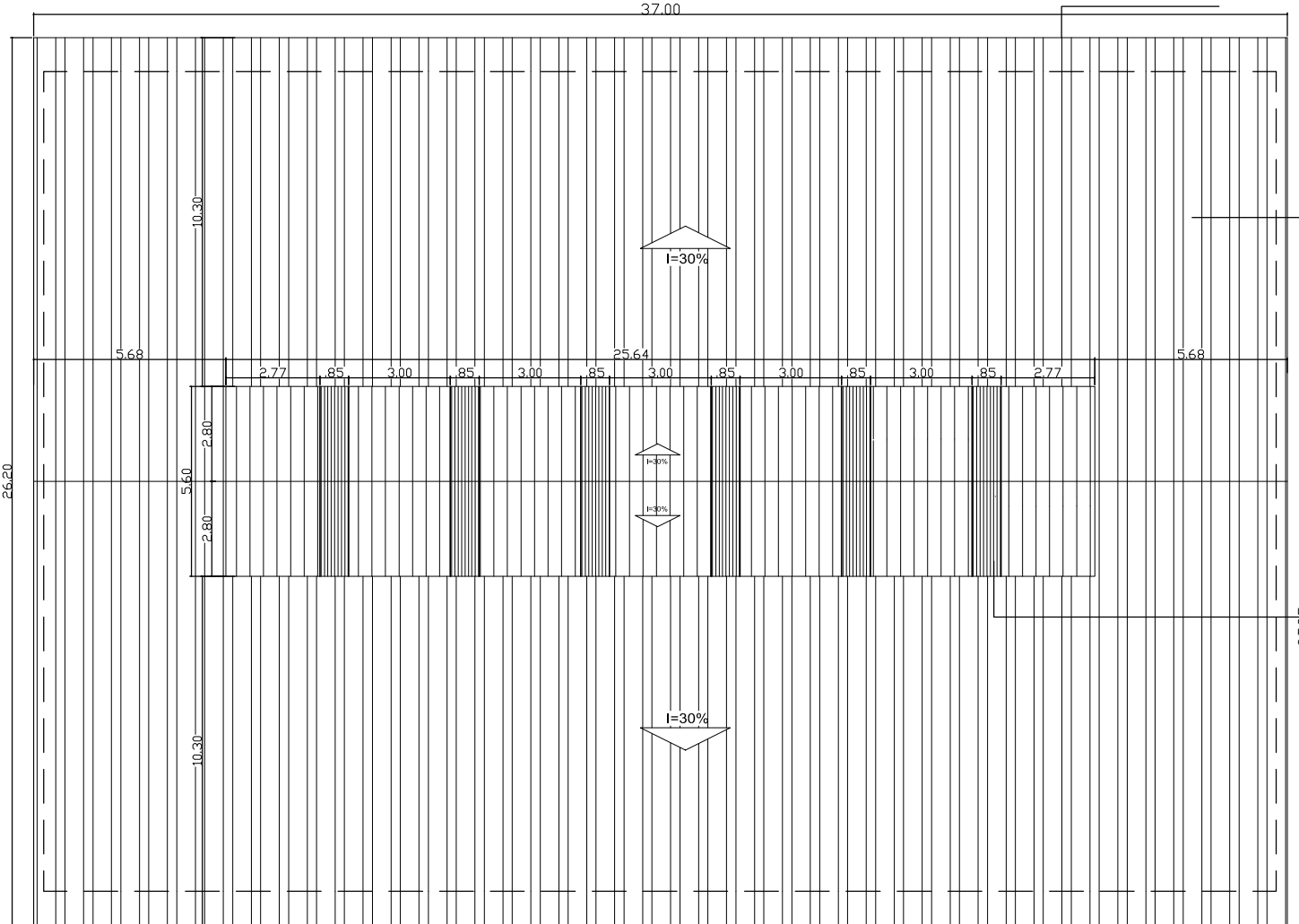
PLANTA DE COBERTURA Esc.: 1/200
