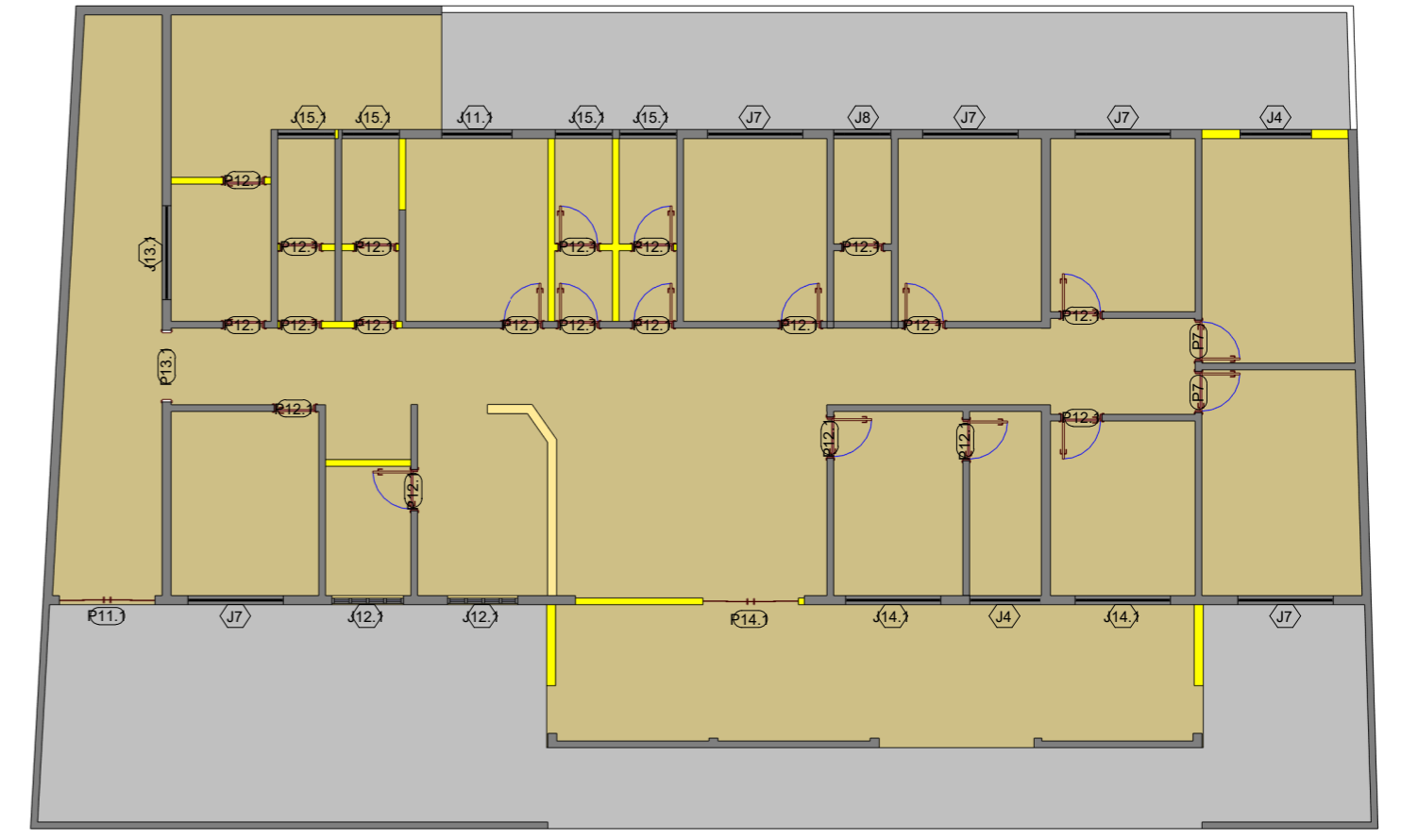
2 PLANTA - TÉRREO DEMOLIÇÃO 1 : 150
