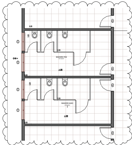
2 PLANTA BAIXA 1:50
