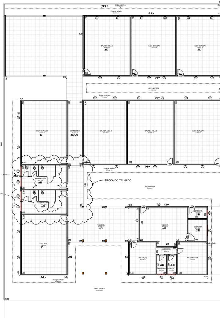
1 PLANTA BAIXA 1:100
