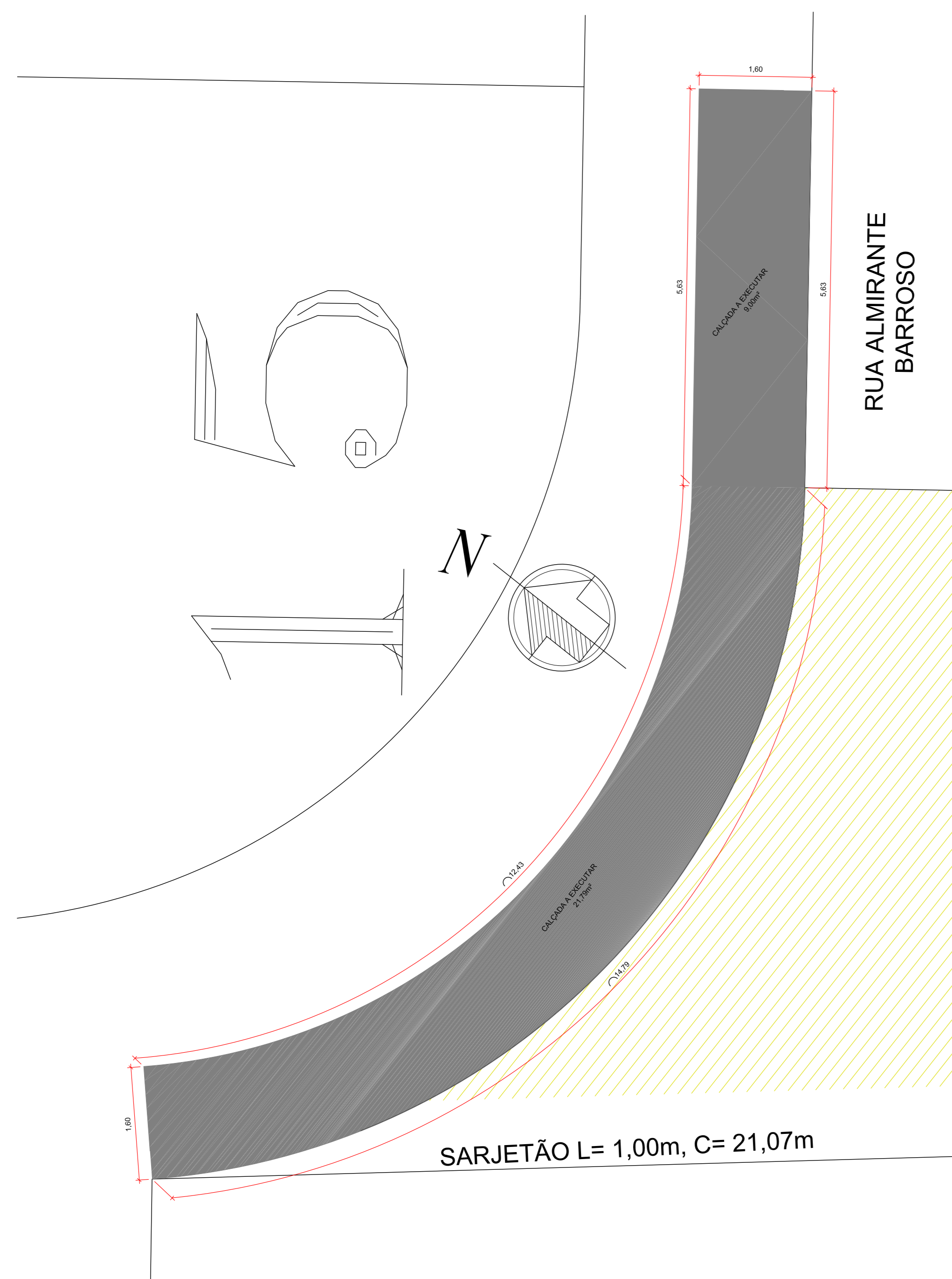
IMPLANTAÇÃO DA CALÇADA- CALÇADA 02 LADO ESQUERDO À JUSANTE DA R. Dª AMÉLINA ESCALA 1:50
