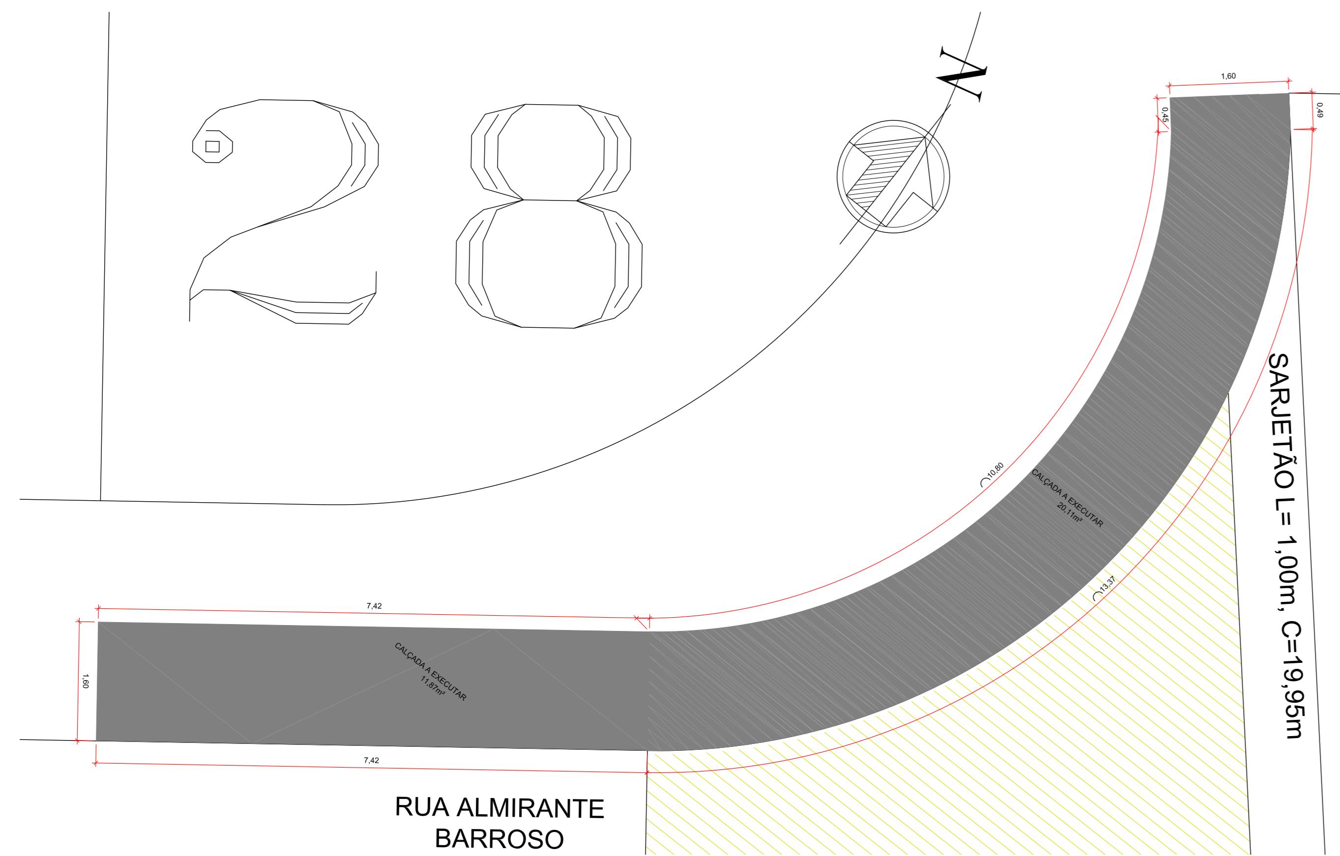
IMPLANTAÇÃO DA CALÇADA- CALÇADA 01 LADO ESQUERDO À JUSANTE DA R. Dª AMÉLINA ESCALA 1:50
