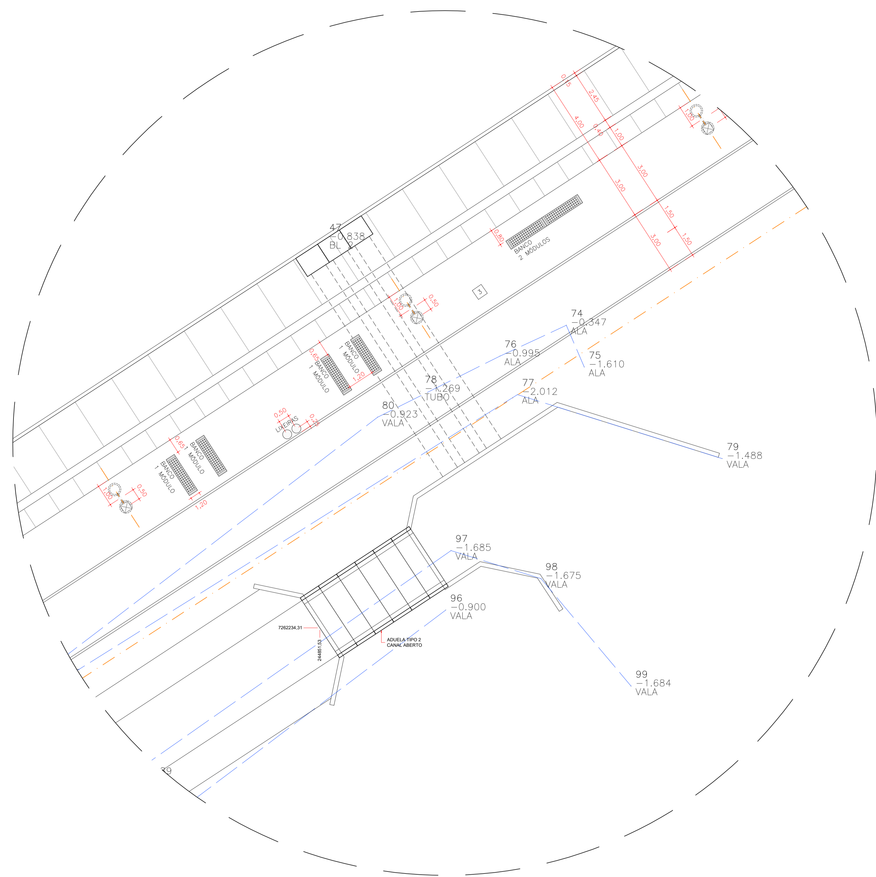
LOCAÇÃO - TRECHO 3 ESCALA 1:100
