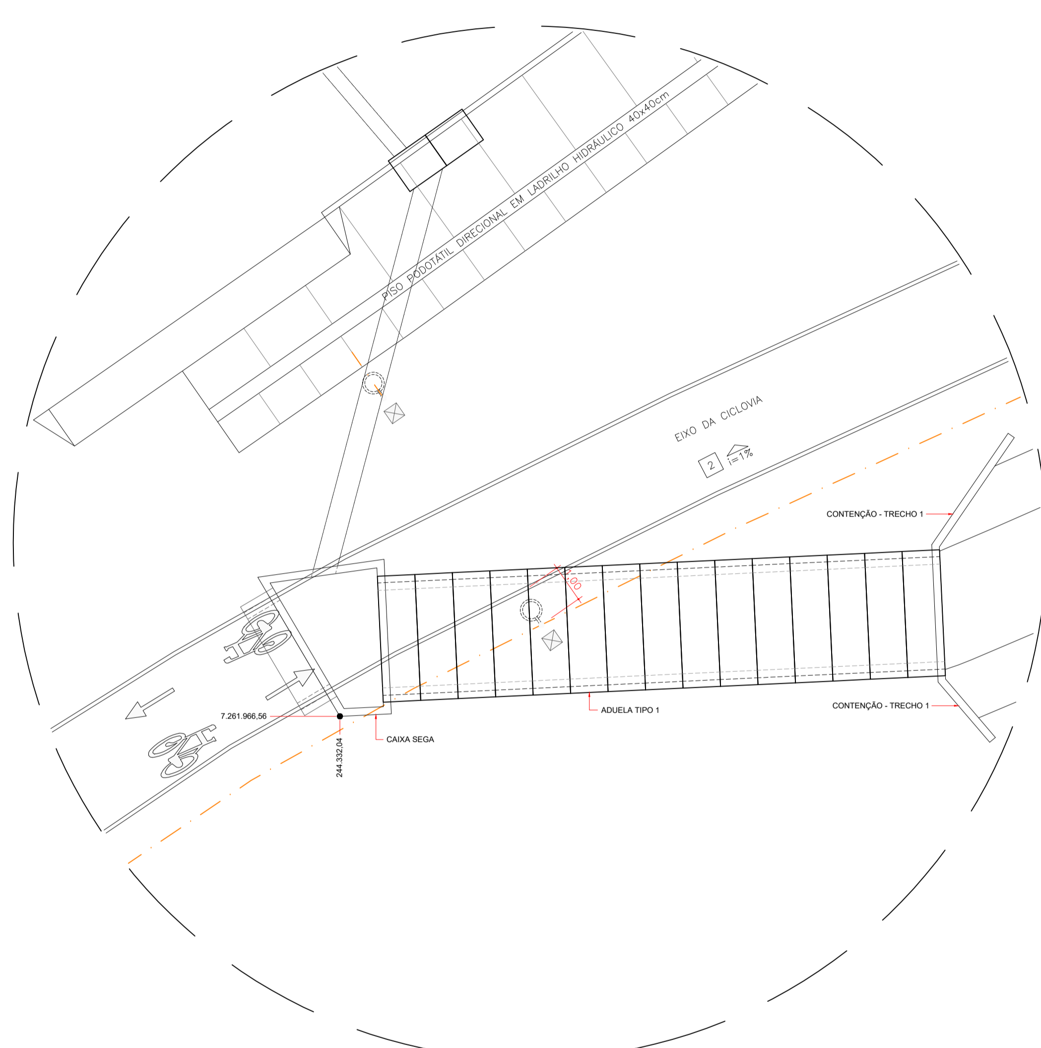
LOCAÇÃO - TRECHO 1 ESCALA 1:100
