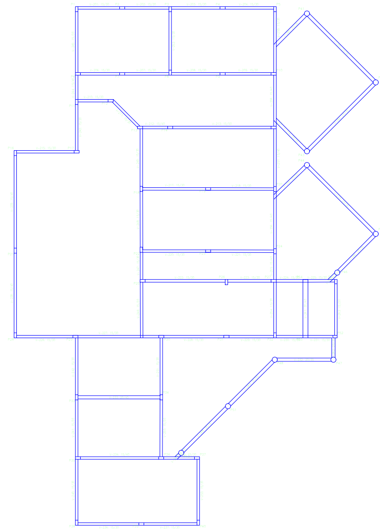
LOCAÇÃO DAS VIGAS ESC. 1/100
