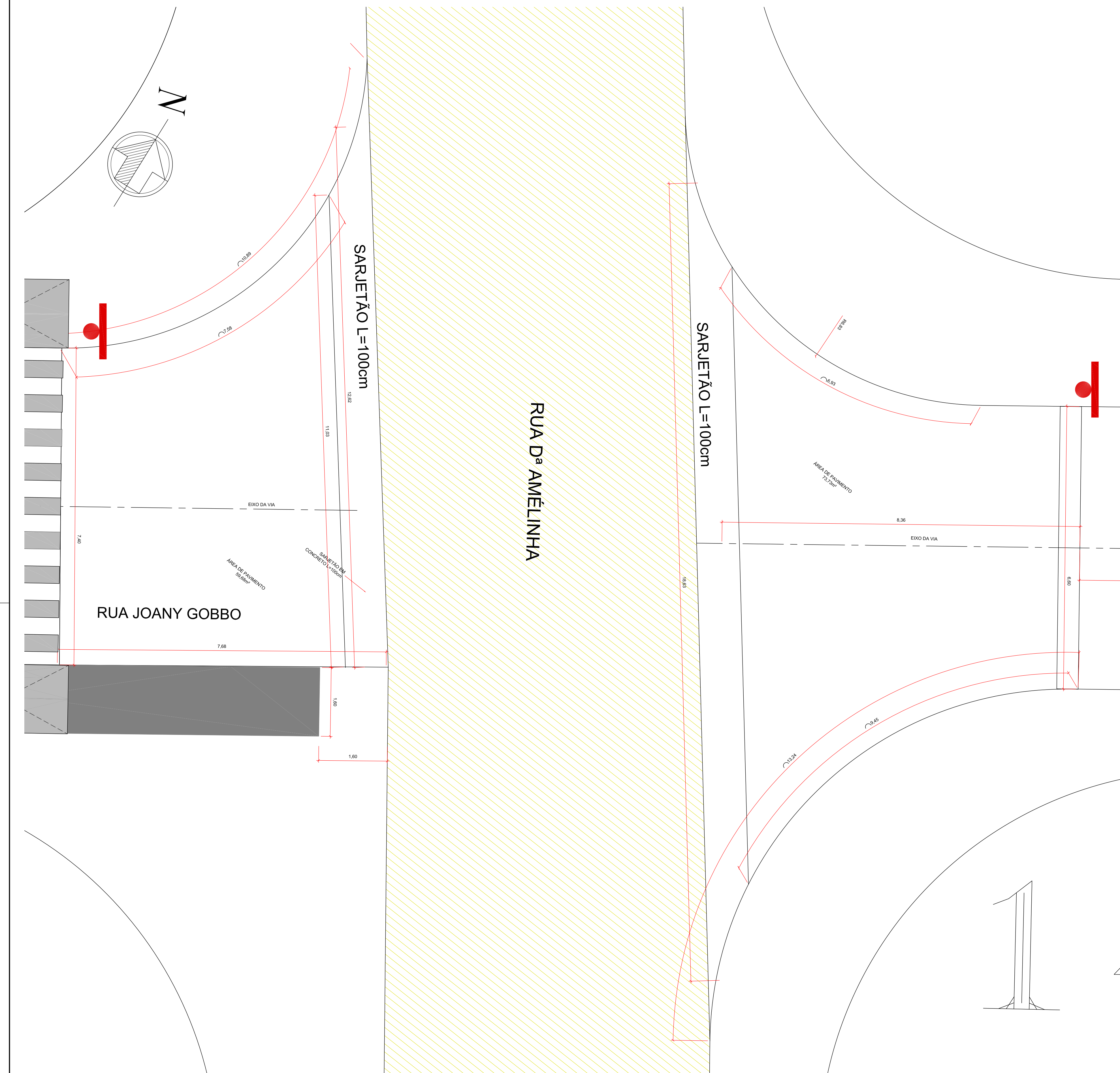
IMPLANTAÇÃO EMBOCADURA - RUA JOANY GOBBO C/ Dª AMELÍNHA ESCALA 1:25
