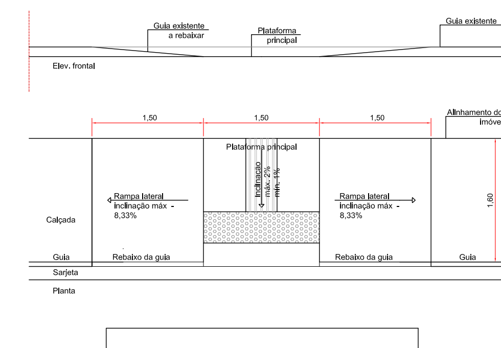
DETALHE RAMPAS DE ACESSIBILIDADE ESCALA 1:25
