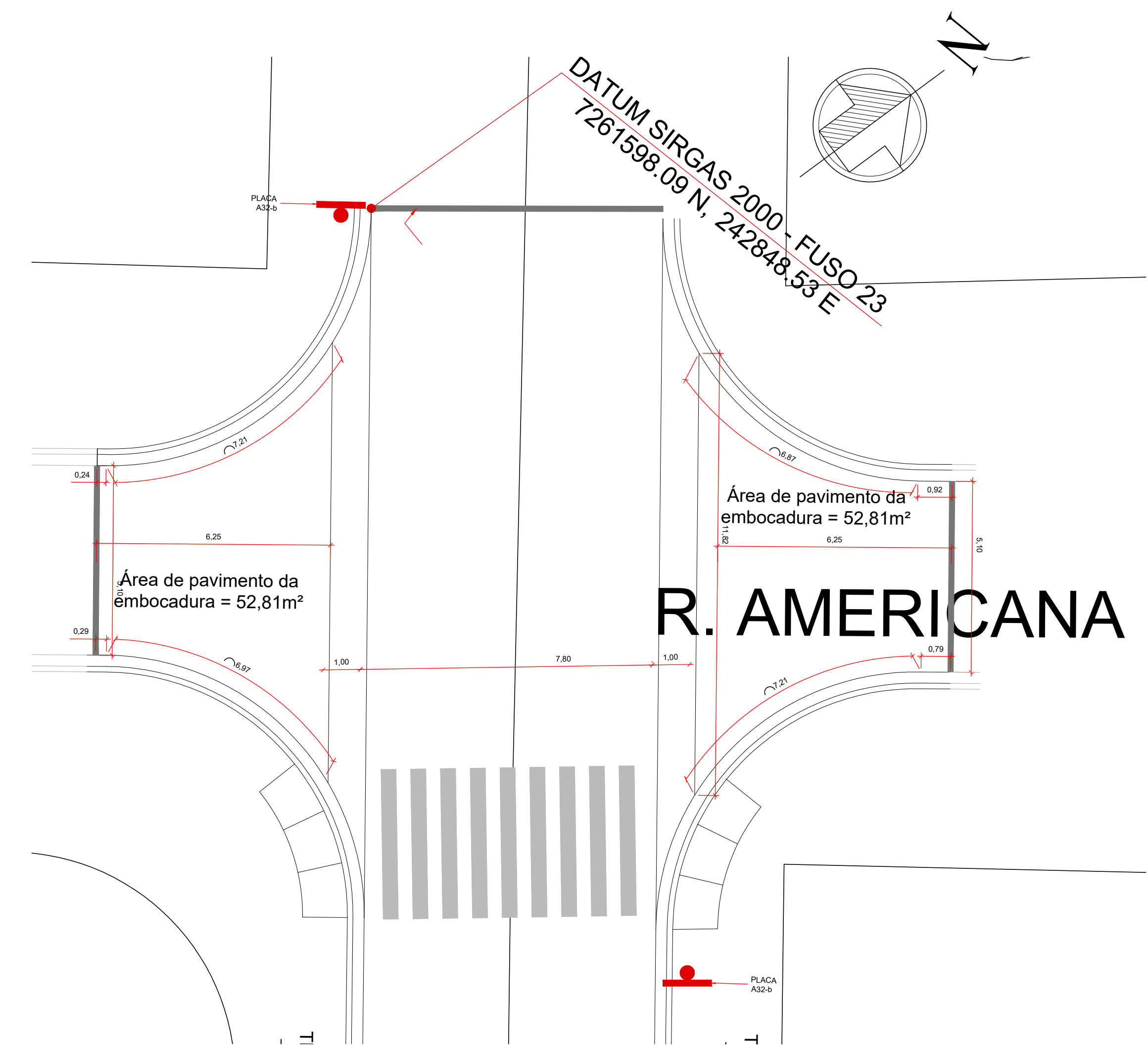
IMPLANTAÇÃO EMBOCADURA - R. SOROCABA C/ RUA AMERICANA ESCALA 1:50
