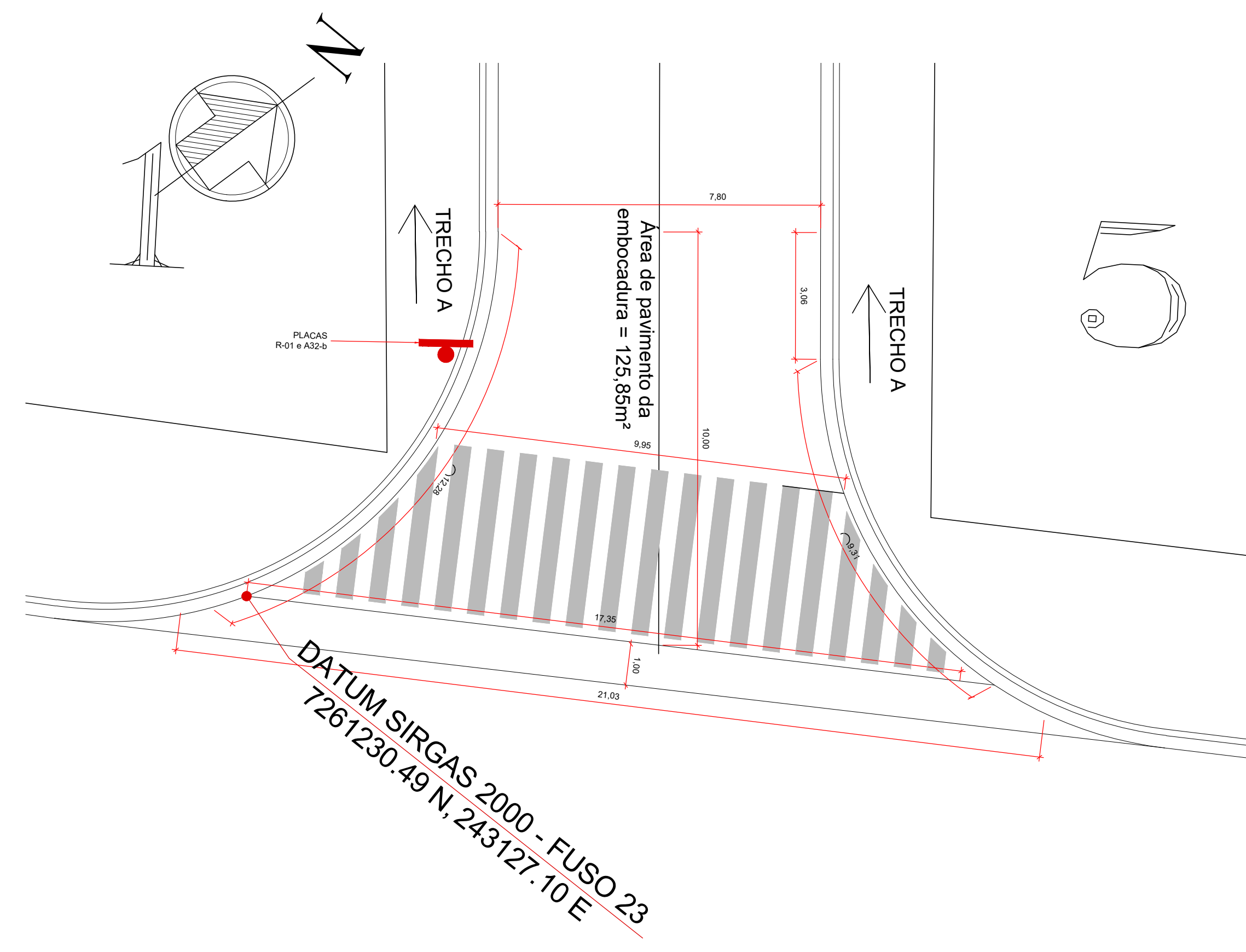
IMPLANTAÇÃO EMBOCADURA - AV. BERA MAR C/ R. SOROCABA ESCALA 1:50
