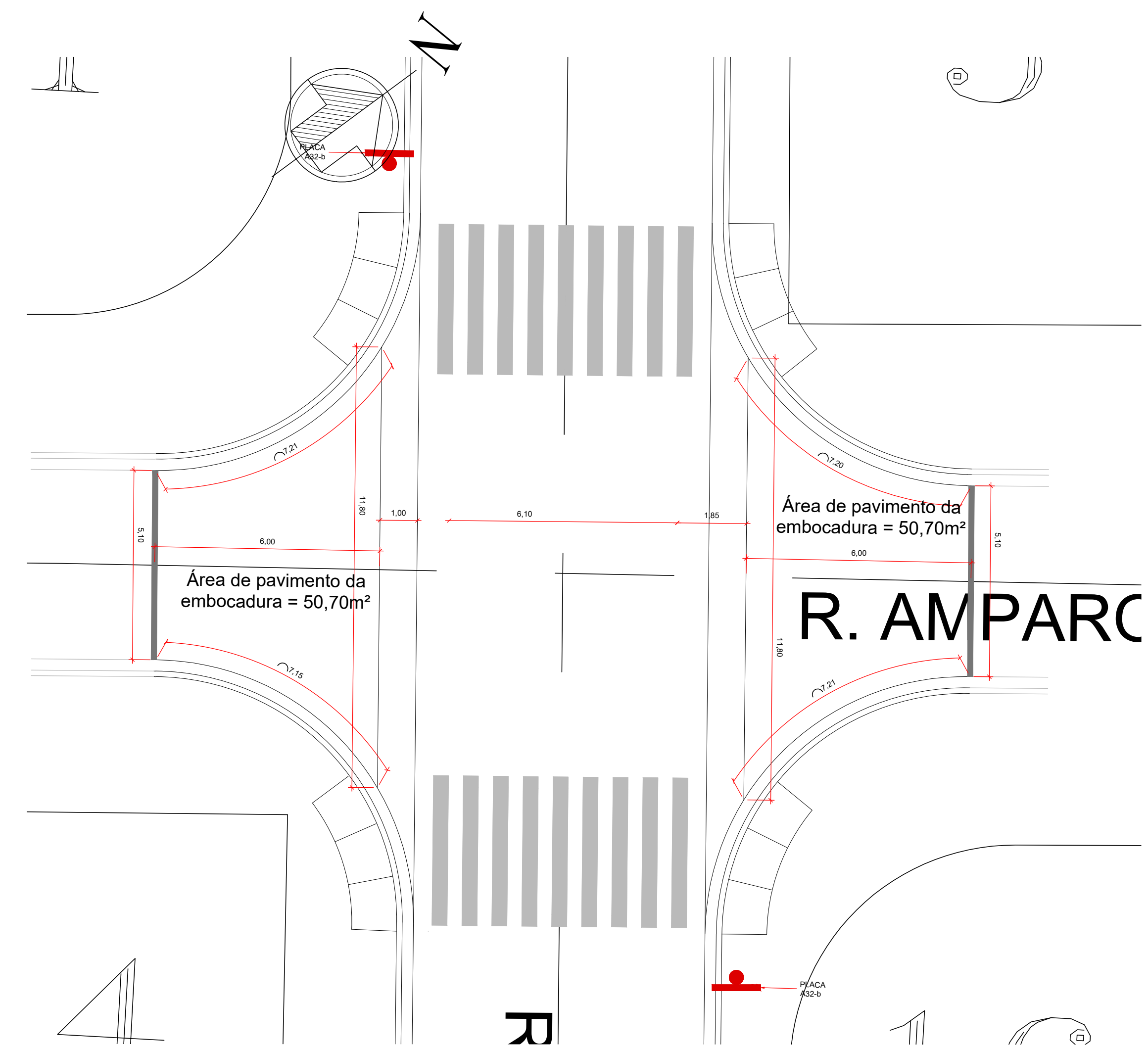
IMPLANTAÇÃO EMBOCADURA - R. SOROCABA C/ RUA AMPARO ESCALA 1:50
