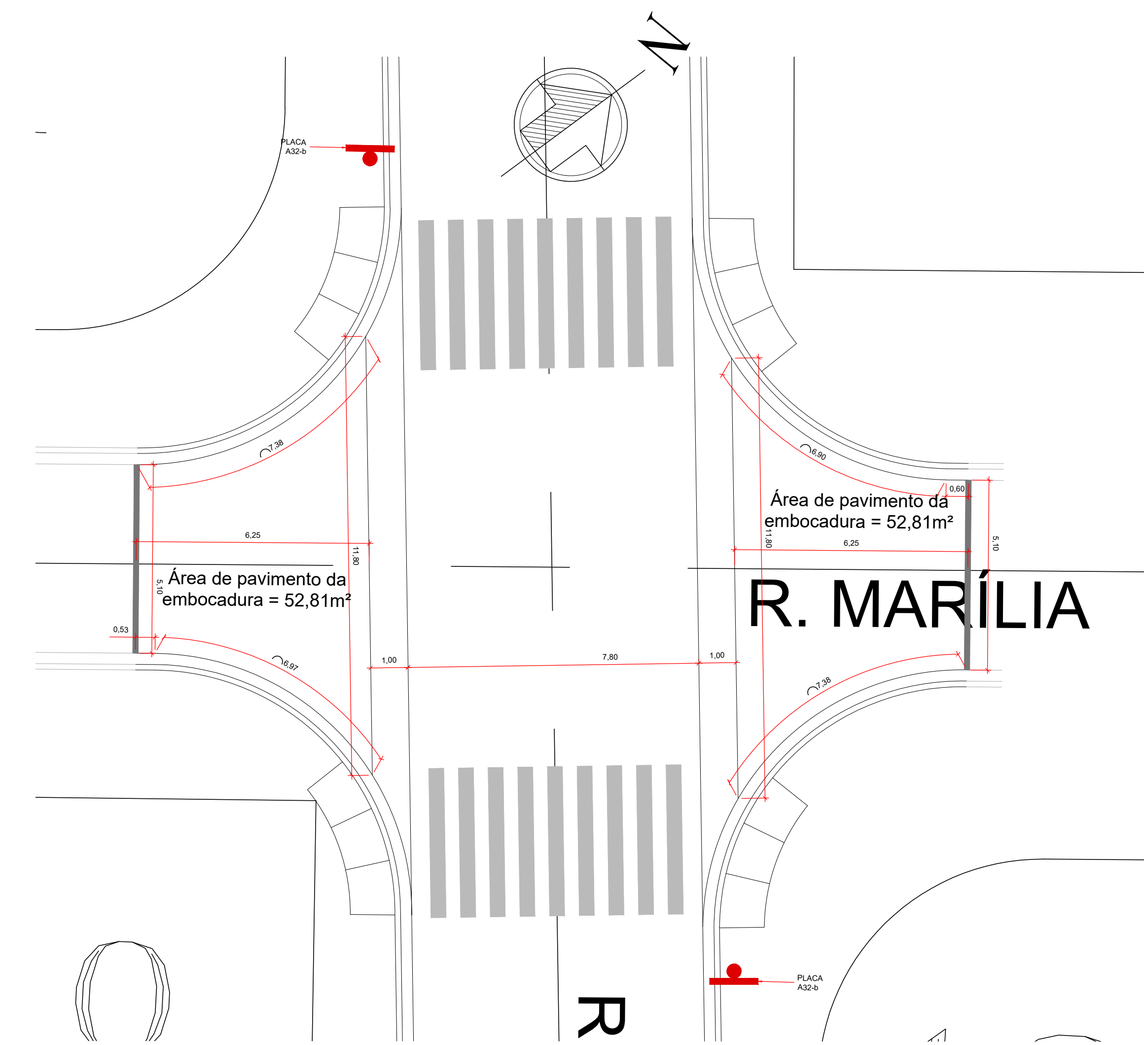
IMPLANTAÇÃO EMBOCADURA - R. SOROCABA C/ RUA MARÍLIA ESCALA 1:50
