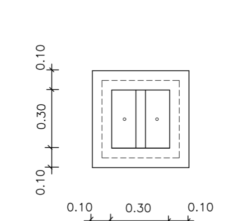
DETALHE DA CAIXA DE GORDURA ESCALA 1/20
