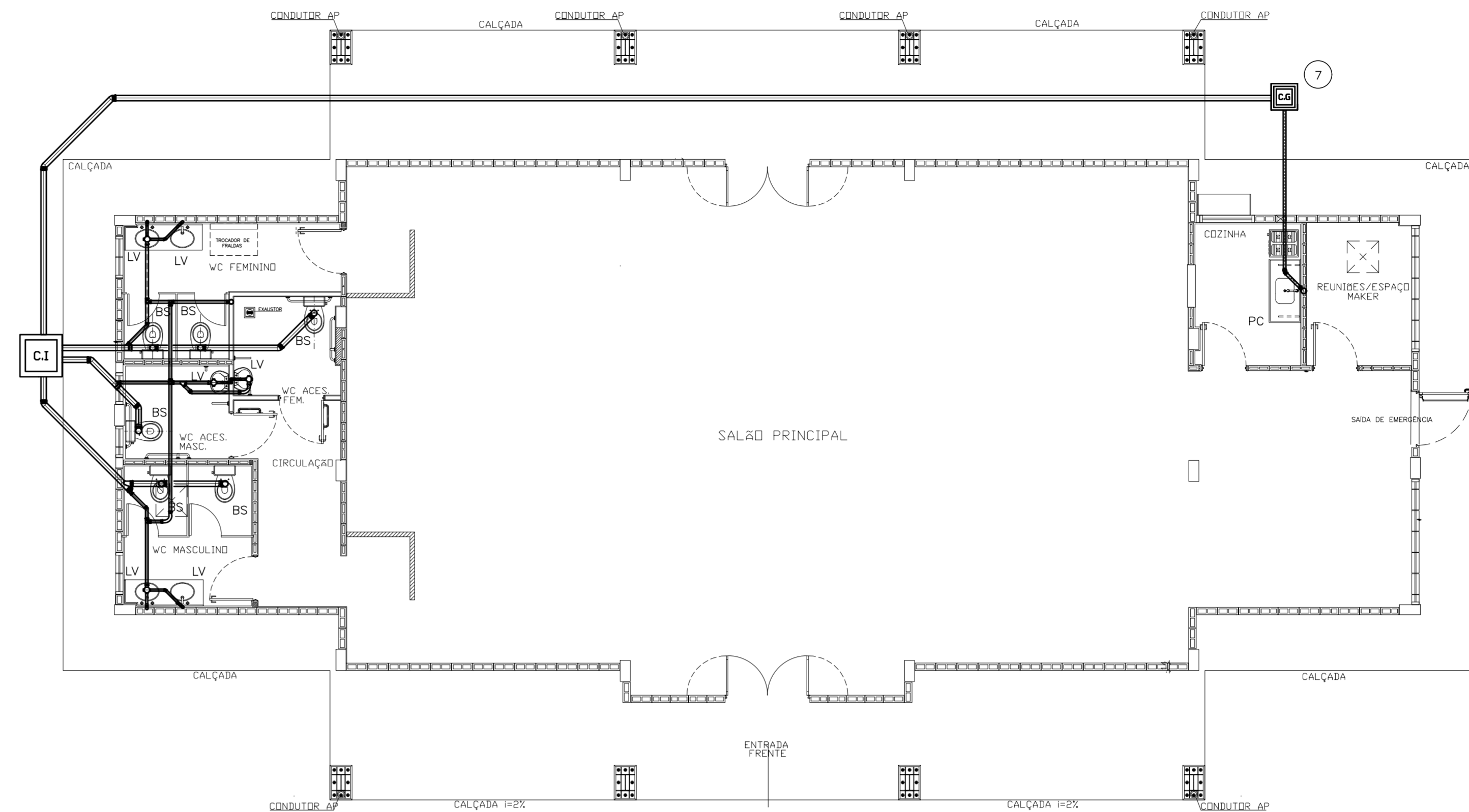
PLANTA DE ESGOTO ESCALA 1/75
