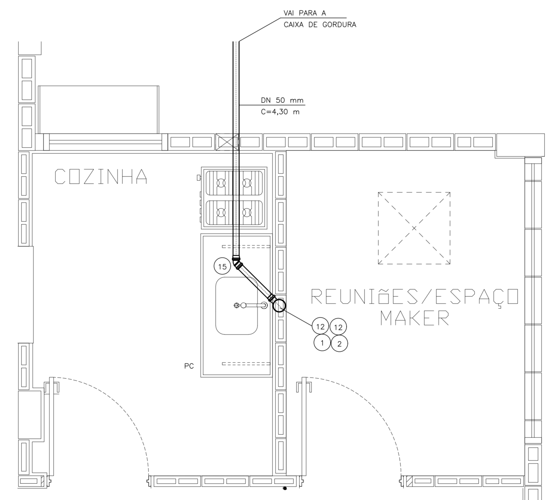
DETALHE DO ESGOTO ESCALA 1/20
