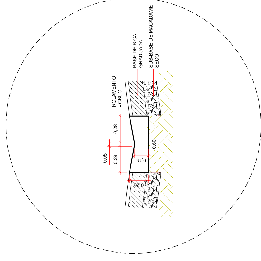
DET. SARJETÃO EMBOCADURA DA RUA ALMIRANTE BARROSO ESCALA 1:25
