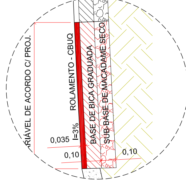
DET. PAV. A RESTAURAR EMBOCADURA AV. BEIRA MAR ESCALA 1:25
