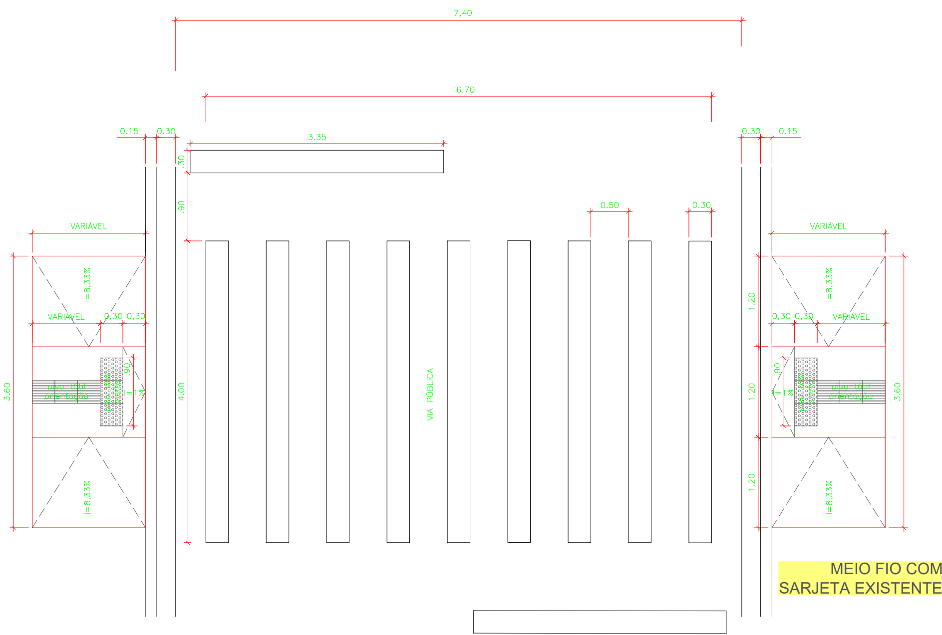
DETALHE 3 – FAIXA DE PEDESTRE
