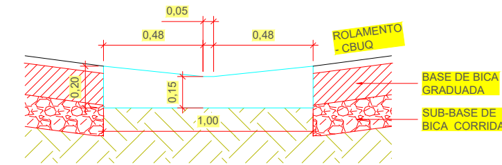
DETALHE 4 – SARJETÃO
