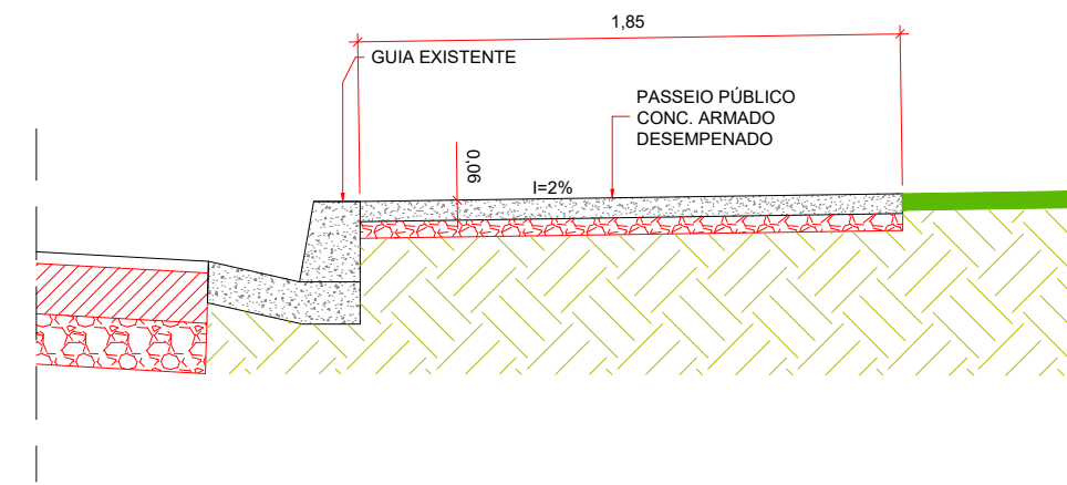
DETALHE 2 – CALÇADA
