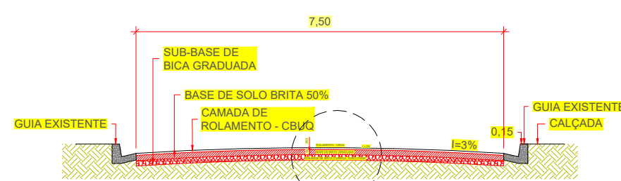
DETALHE 5 – SEÇÃO TRANSVERSAL DO PAVIMENTO
