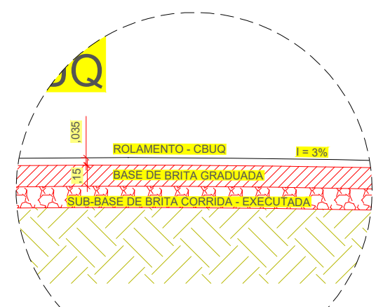
DETALHE DO PAVIMENTO – CAMADAS
