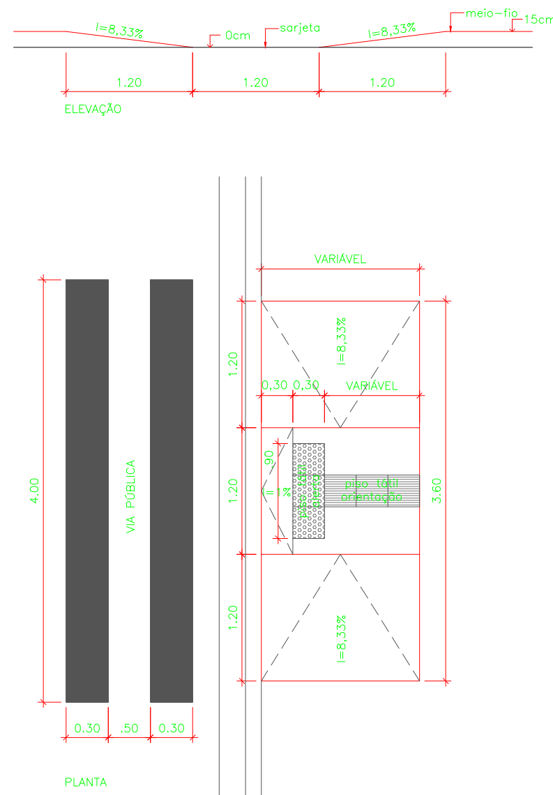
DETALHE 1 – RAMPA DE ACESSIBILIDADE
