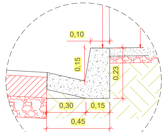
DETALHE 6 – GUIA E SARJETA
