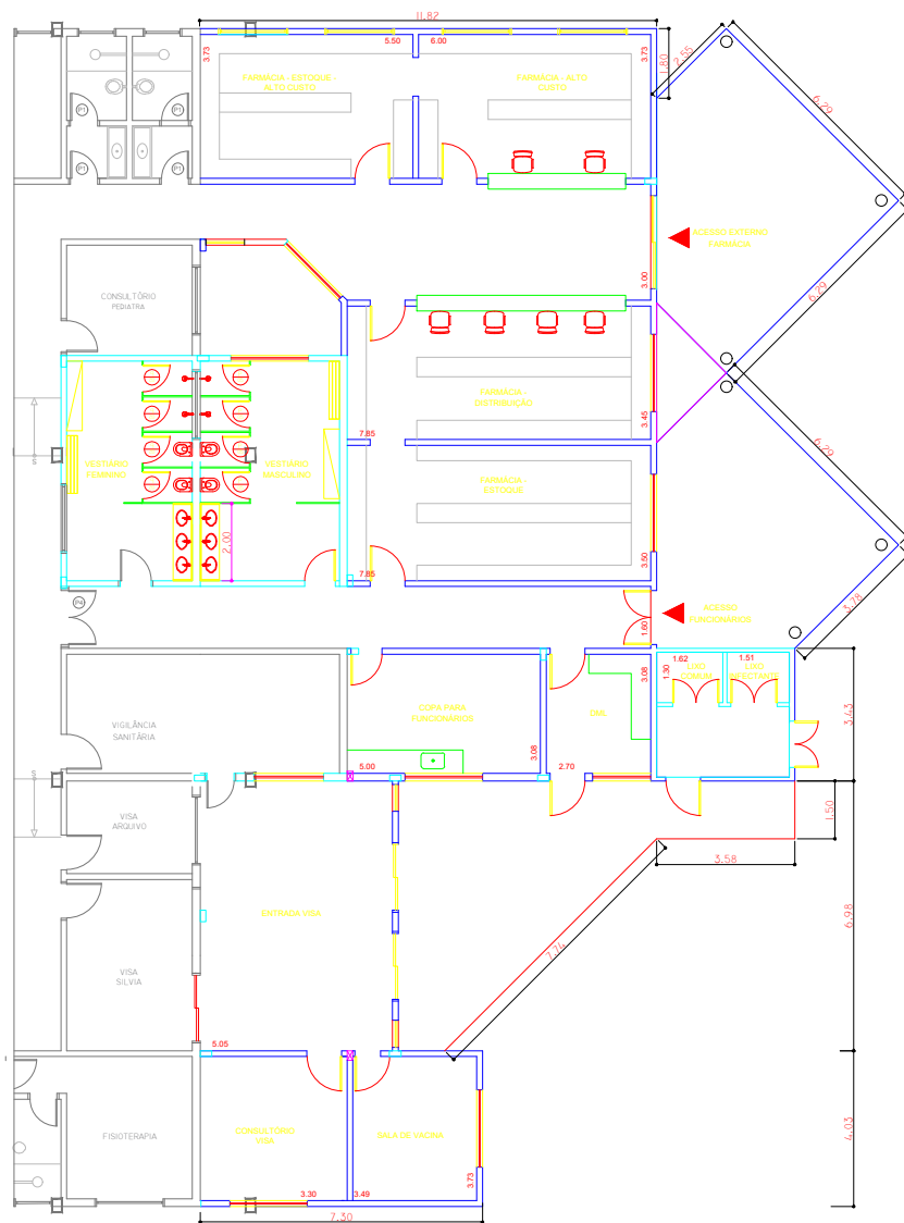
PLANTA BAIXA DE AMPLIAÇÃO ESC. 1/100
