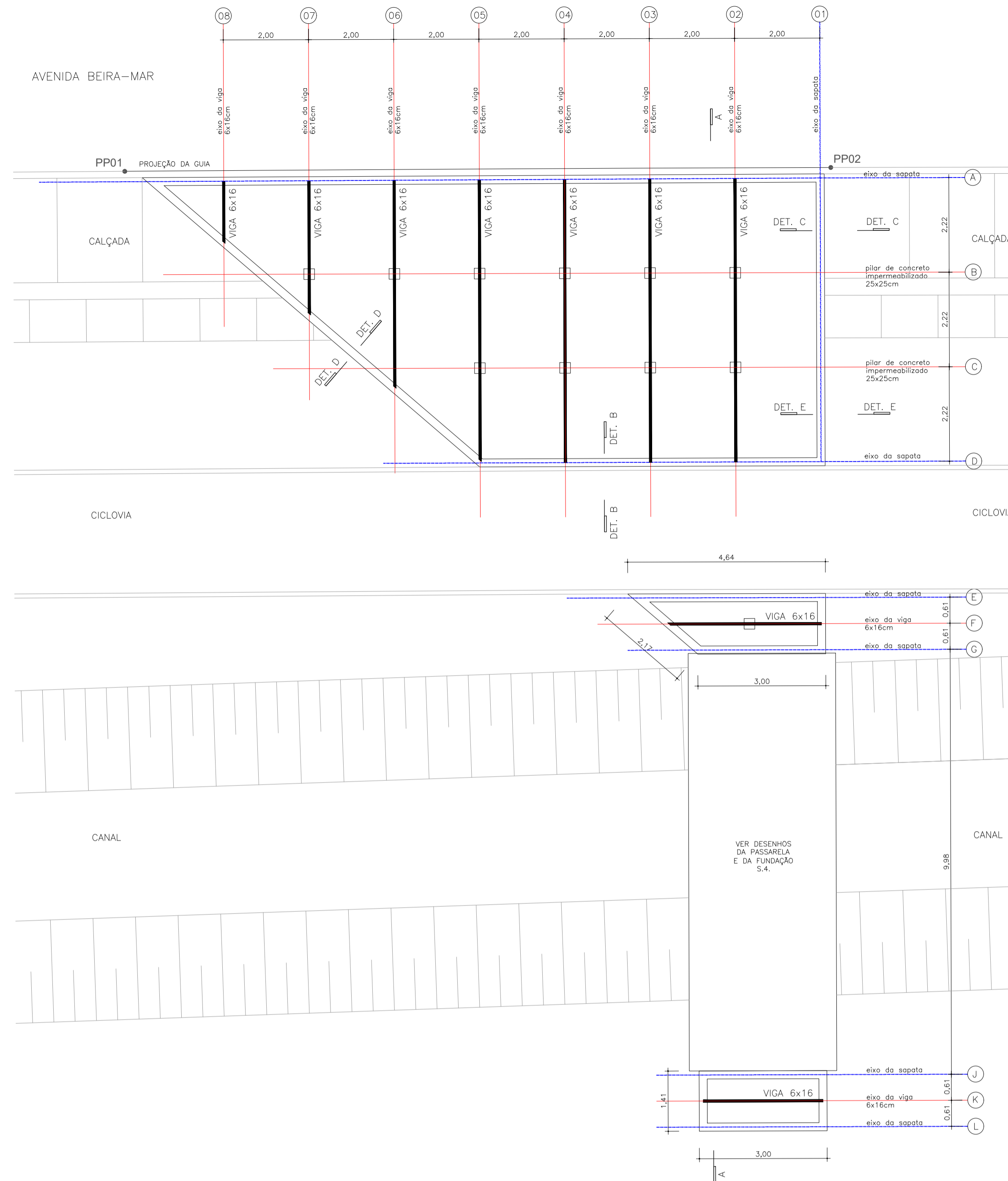
PLANTA DE VIGAMENTO DO DECK ESCALA 1:75
