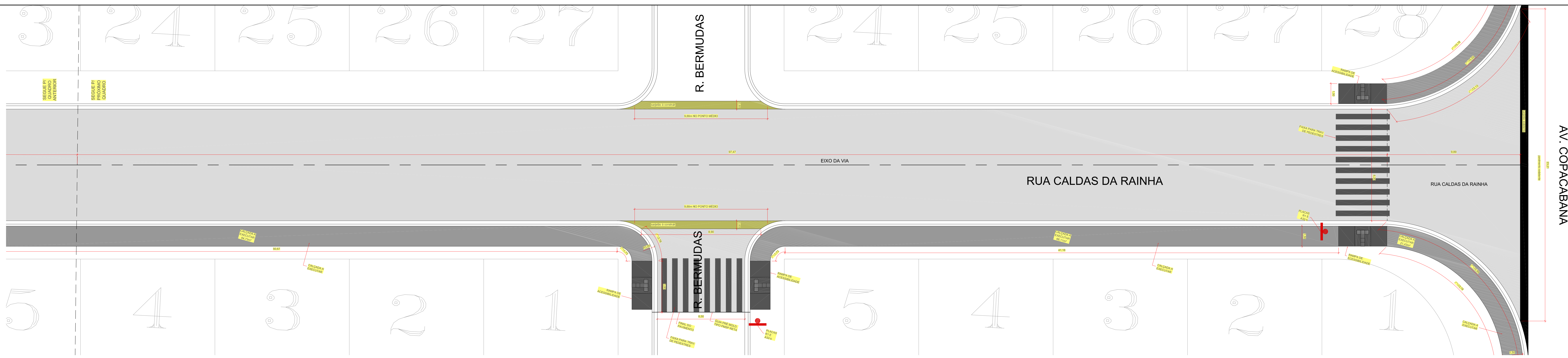
PLANTA DE PAVIMENTAÇÃO – PRIMEIRO TRECHO ESCALA 1:100
