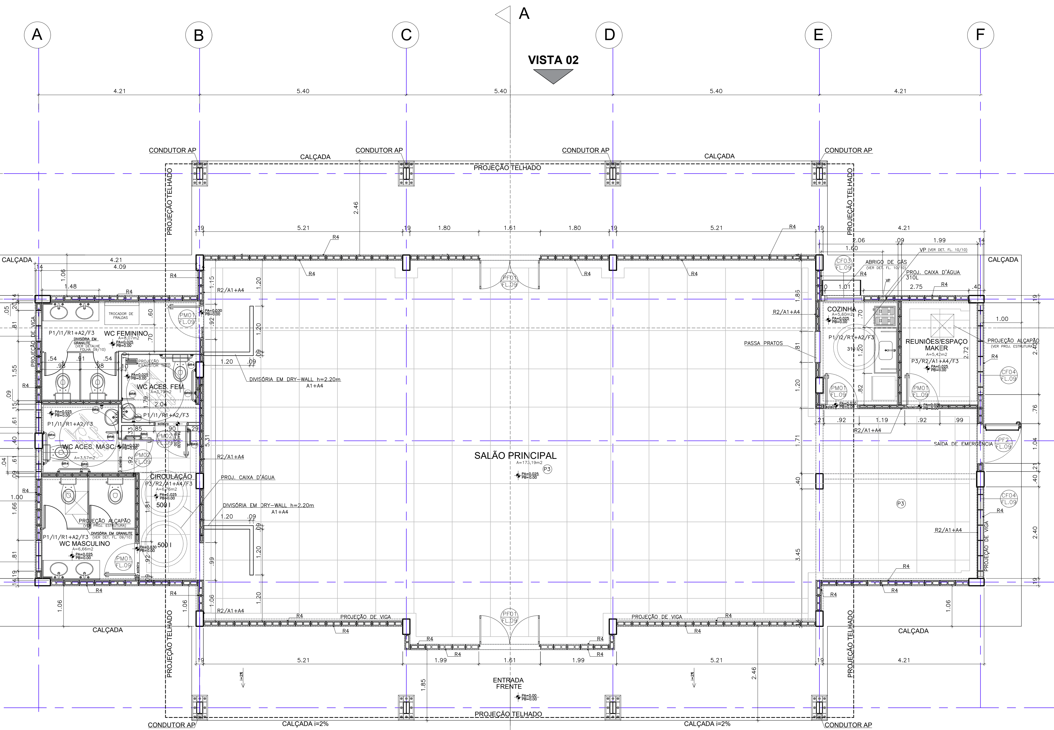
PLANTA ESC.: 1:50
