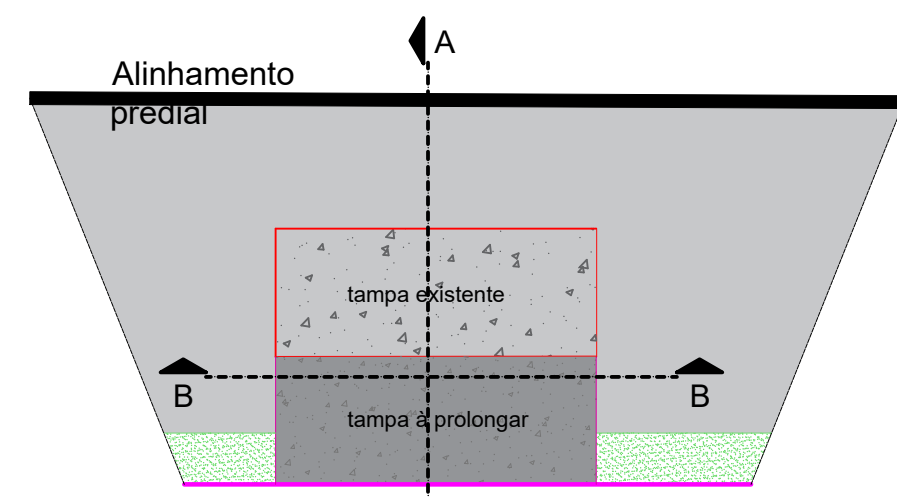
DETALHE BOCA DE LOBO escala:: 1:250
